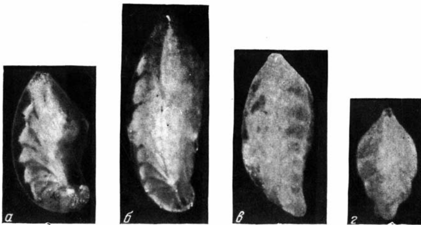
Рис. 2. Изменение числа камер в начальной части раковины Saracenaria pravoslavlevi Furss. et Pol. и образование переходных форм от рода Saracenaria к роду Tristix .
