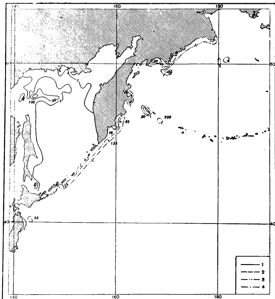
Рис. 17. Распространение в северо-западной части Тихого океана
