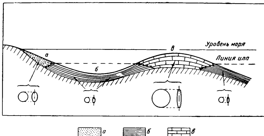
Распределение нуммулитов различных размеров в отложениях неритовой зоны а — песчаные отложения сублиторали с выпуклыми нуммулитами средних размеров; б — глины псевдоабиссали с мелкими тонкими нуммулитами; в — известняки мелководной области открытого моря с крупными дисковидными нуммулитами.
