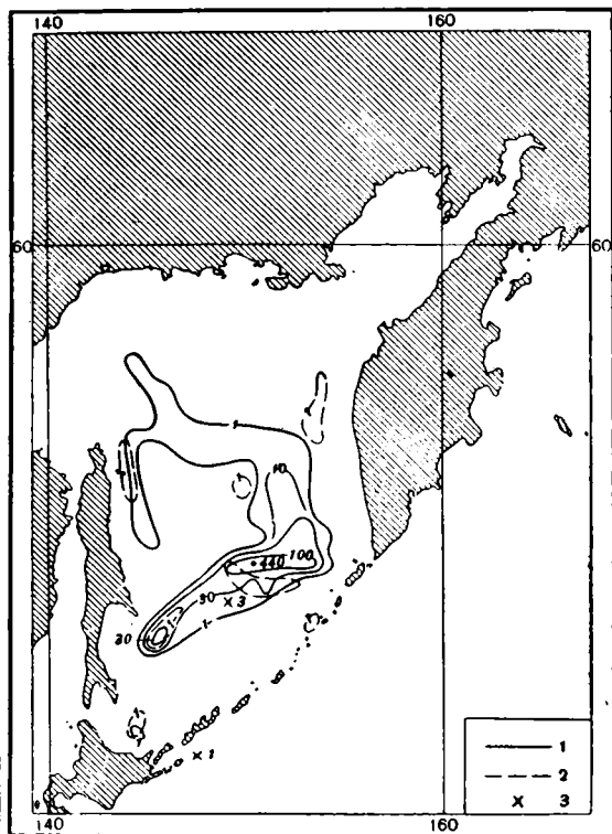
Рис. 20. Распространение в северо-западной части Тихого океана 1 — Bolivina subspinescens ; 2 — B. seminuda и 3 — B. alata (в экземплярах на 50 г осадка)
