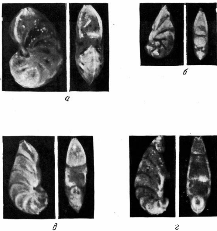
Рис. 10. Изменение формы раковины и переход их по типу строения от рода Lenticulina к роду Saracenaria .
