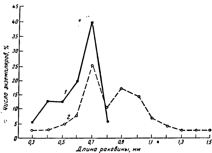
Рис. 7. Кривые изменения длины раковин
