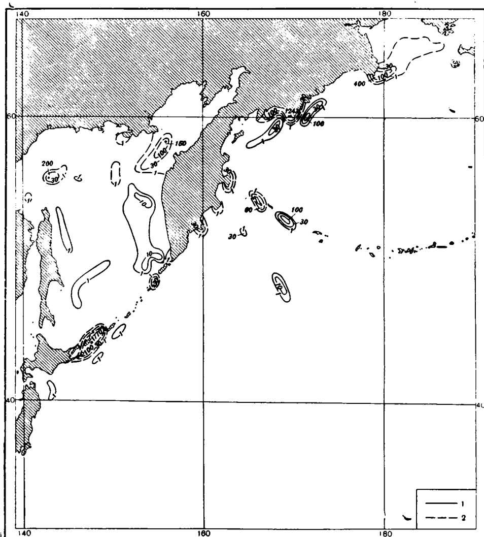
Рис. 4. Распространение в северо-западной части Тихого океана 1 — Cibicides pseudoungerianus и 2 — Dyocibicides biserialis (в экземплярах на 50 г осадка)
