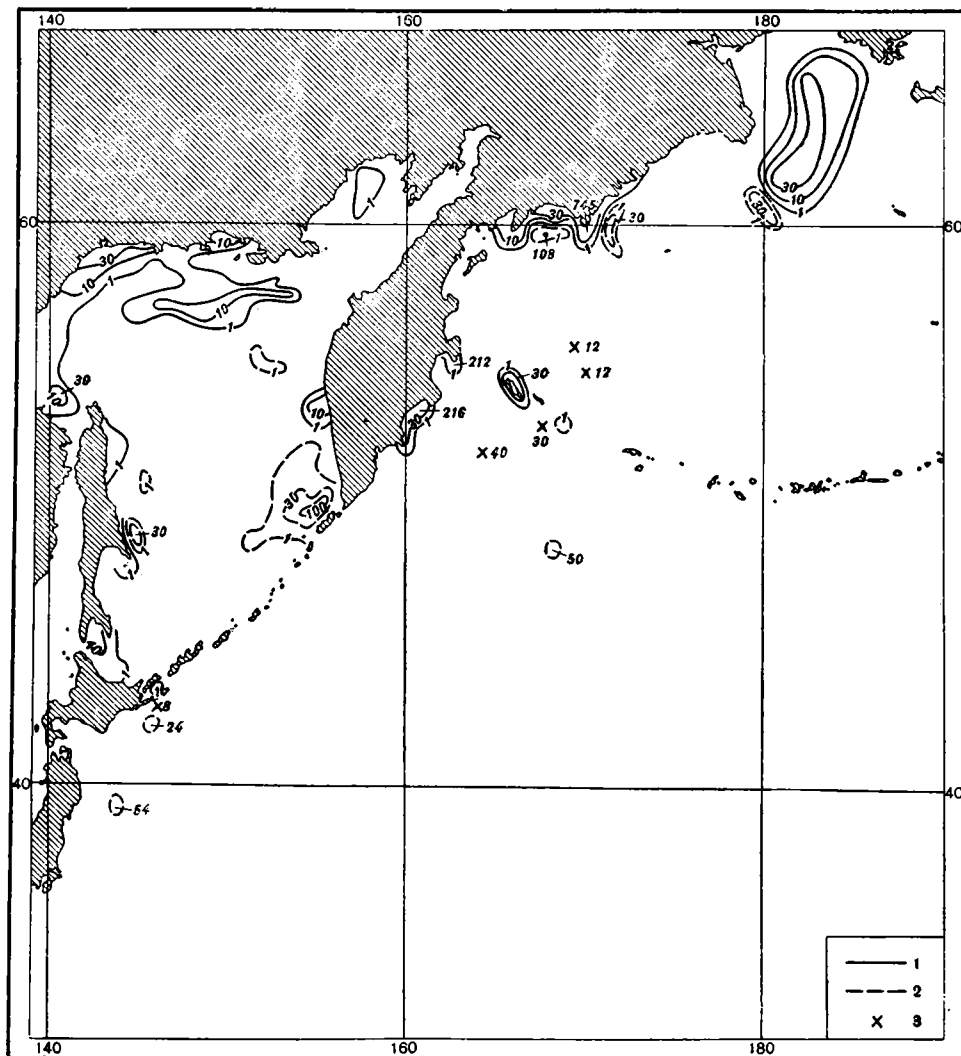
Рис. 7. Распространение в северо-западной части Тихого океана
