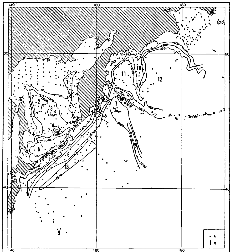
Рис. 1. Карта станций и биометрическая схема северо-западной части Тихого океана а — место взятия проб; б — основные геоморфологические элементы дна; 1 — котловина ТИНРО; 2 — котловина Дерюгина; 3 — возвышенность Института океанологии; 4 — возвышенность Академии наук СССР; 5 — южная глубоководная котловина Охотского моря; 6 — Курило-Камчатская глубоководная впадина; 7 — возвышенность Обручева; 8 — Гавайский хребет; 9 — гора Исакова; 10 — хребт Ширшова; 11 — западная глубоководная котловина Берингова моря; 12 — восточная глубоководная котловина Берингова моря; 13 — возвышенность Зенкевича; 14 — Алеутская глубоководная впадина
