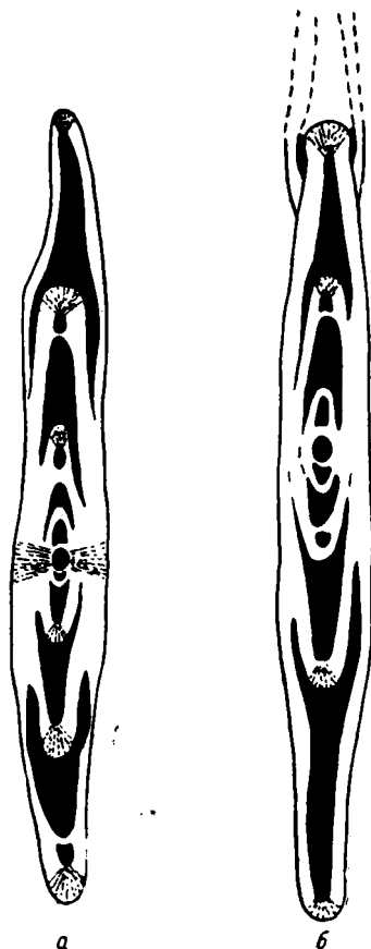
Рис. 2. Neooperculinoides orbigny (Galeotti) (A)
