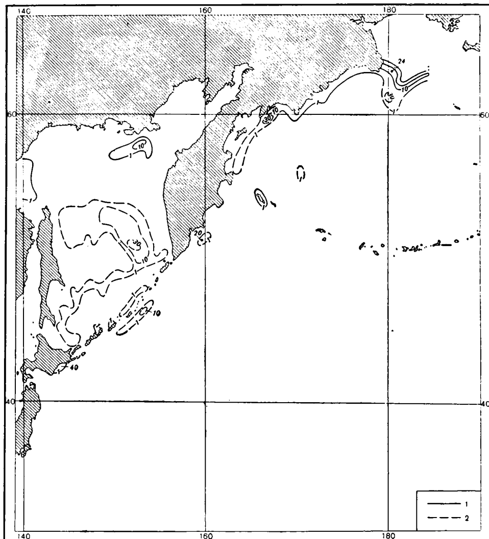
Рис. 12. Распространение в северо-западной части Тихого океана 1— Globobulimina auriculata orbiculata и 2— G. auriculata elongata (в экземплярах на 50 г осадка)
