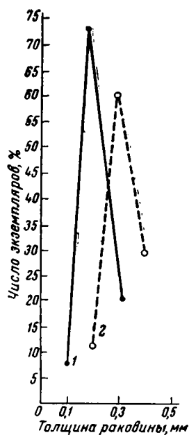
Рис. 6. Кривые изменения толщины раковин
