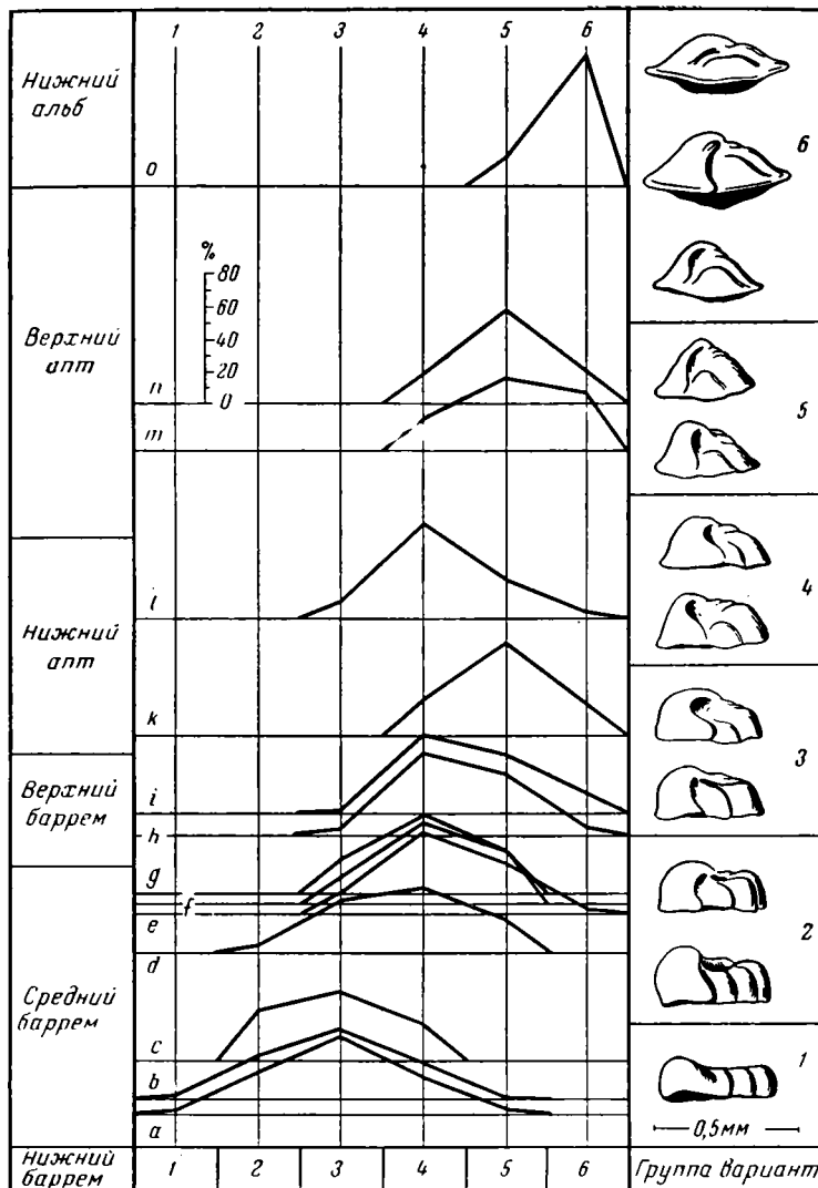
Рис. 2. Вариационные кривые изменчивости Globorotalites bartensteini (Bettenstaedt, 1958).
