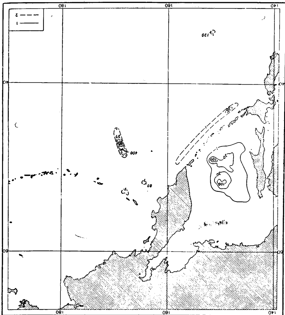
Рис. 14. Распространение в северо-западной части Тихого океана — Uvigerina aueriana ochotica и 2 — U. aueriana complanata (в экземплярах на 50 г осадка)
