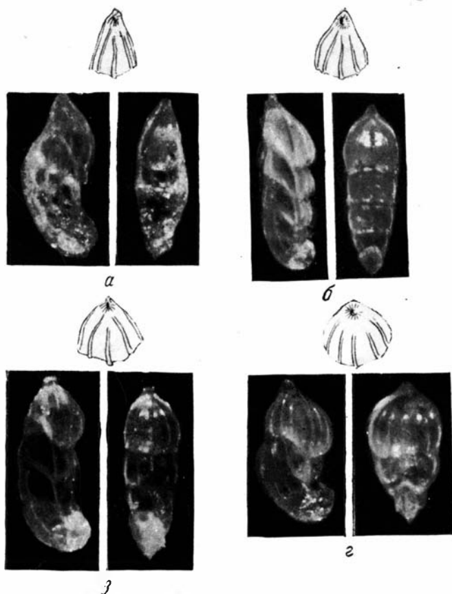
Рис. 9. Изменение формы поперечного сечения раковин Saracenaria mirabilissima Furss. et Pol. и образование переходных форм от рода Saracenaria к роду Marginulina .
