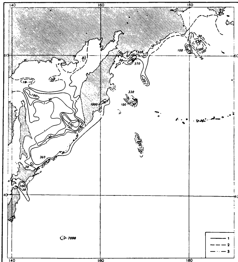
Рис. 13. Распространение в северо-западной части Тихого океана
