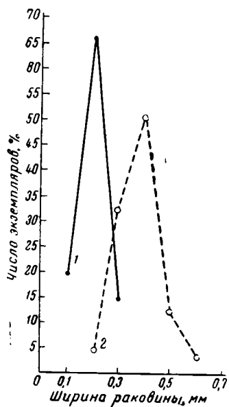
Рис. 5. Кривые изменения ширины раковин
