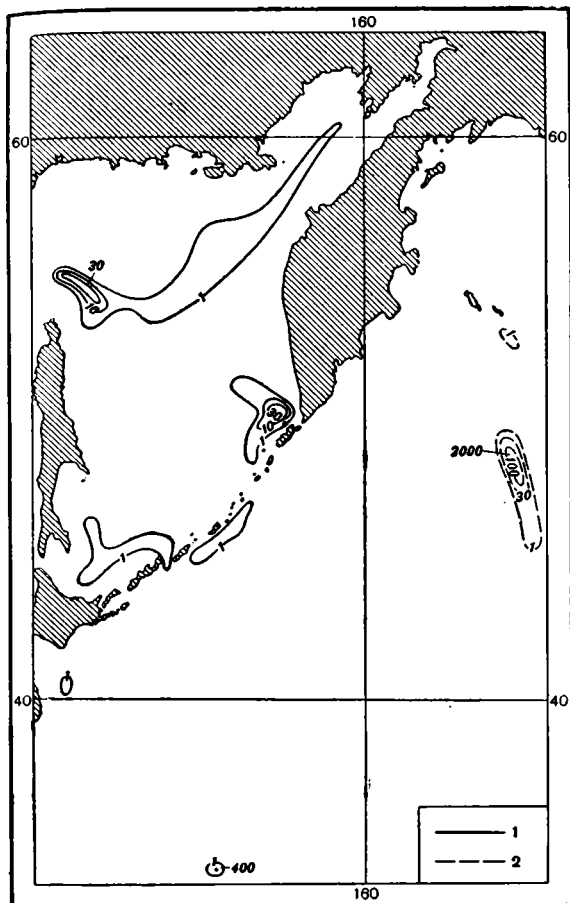
Рис. 19. Распространение в северо-западной части Тихого океана 1 — Bolivina decussata ; 2 — B. spissa и на глубине 400 м — B. quadrilatera (в экземплярах на 50 г осадка)
