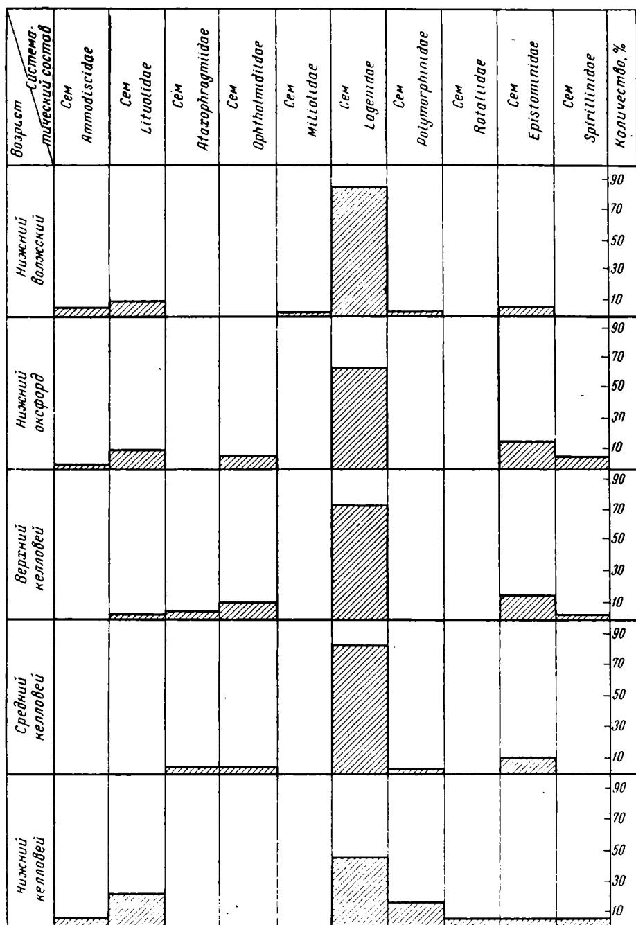
Рис. 1. Диаграмма, показывающая количественные соотношения различных семейств в комплексах верхнеюрских фораминифер Саратовского Поволжья
