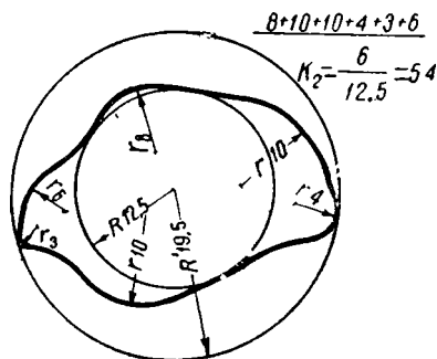
Фиг. 5. Наибольшая вписанная и наименьшая описанная окружности в изображении гальки.
