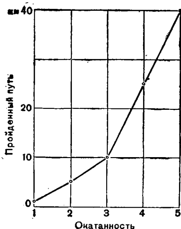
Фиг. 4. — Кривая зависимости окатанности кварцевой гальки от пройденного пути.
