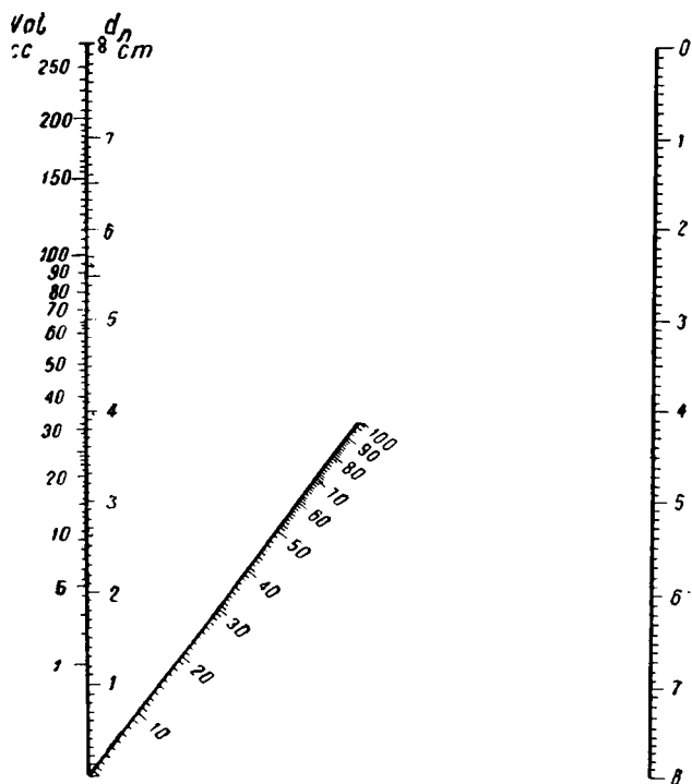
Фиг. 3. — Номограмма Уэйделла.
