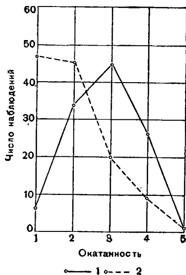
Фиг. 1. — Распределение по классам окатанности гальки кварцита и кварца:
