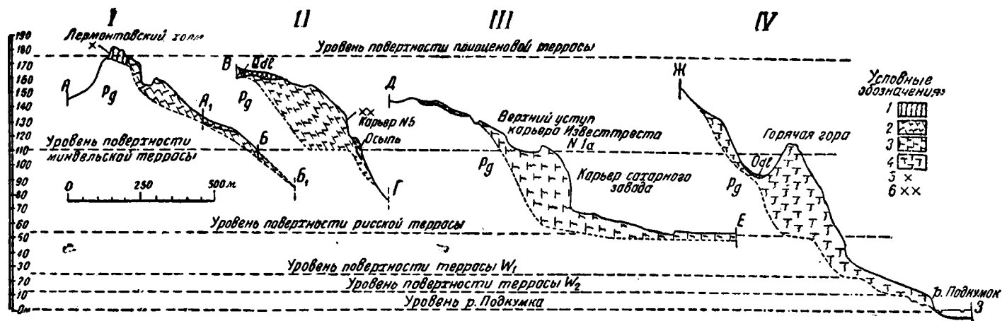
Фиг. 2. Схематические разрезy четырех разновозрастных травертиновых комплексов по склонам Машука и их высотные соотношения с террасами Подкумка.
