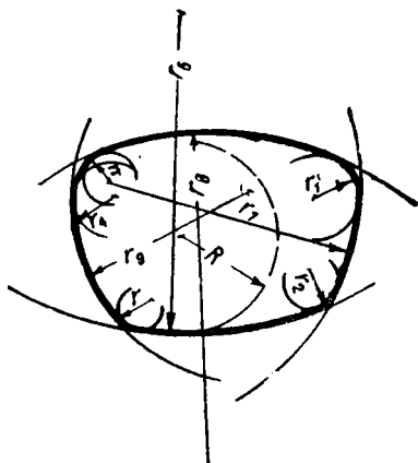
Фиг. 2. Различные радиусы кривизны гальки.
