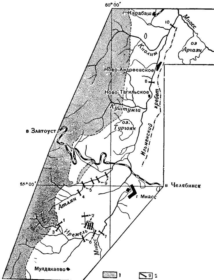
Фиг. 3. — Карта верхнего течения бассейна р. Миасс с показанием распространения свиты «М» и пунктов наблюдения окатанности. Масштаб 1 : 500 000.
