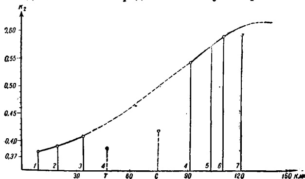
Фиг. 7. Графическое изображение степени обработки речной гальки. Названия пунктов соответствуют №№ на обзорной карте.
