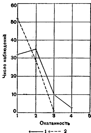
Фиг. 2. — Распределение по классам окатанности гальки массивных и сланцеватых пород:
