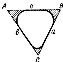
Фиг. 1. Степень окатанности гальки по Тестеру и Бэю.
