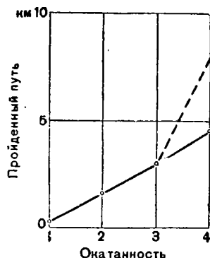
Фиг. 5. — Кривая зависимости окатанности гальки порфирита от пройденного пути.
