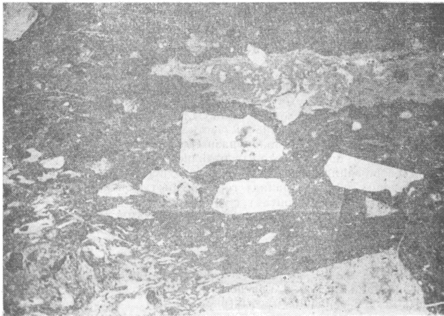
Рис. IV—21. Литонидный игниспумит ескульского типа. Обломки полевых шпатов и фьямме в основной, частично пепловой массе. Ув. 22, при одном никеле.
