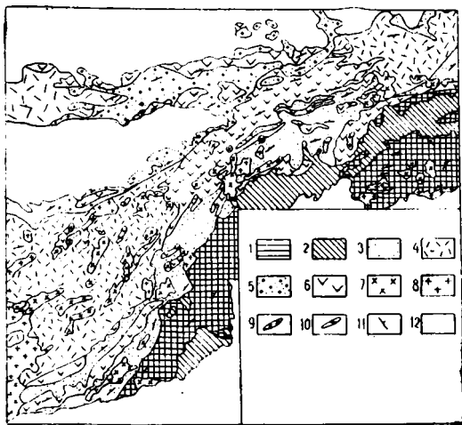
Рис. 11—12. Схема геологического строения андезитовых стратовулканов в горах Матай и Дигерес (геологическая основа В. В. Науменко).
