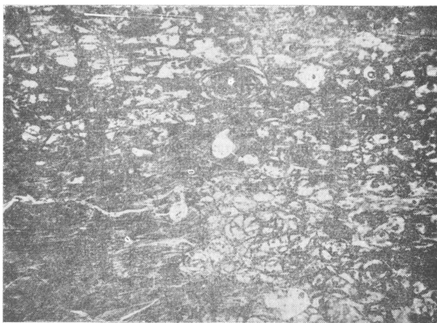
Рис. IV—6. Стекловатый игнимбрит архарлинского типа. Перлитовая текстура (микроотдельность) основной массы. Ув. 45, при одном николе.
