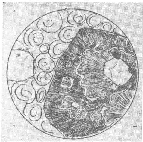
Рис. XIII—8. Вулканическое стекло с перлитовой текстурой и крупными сферолитами. Ув. 22, при одном никеле.
