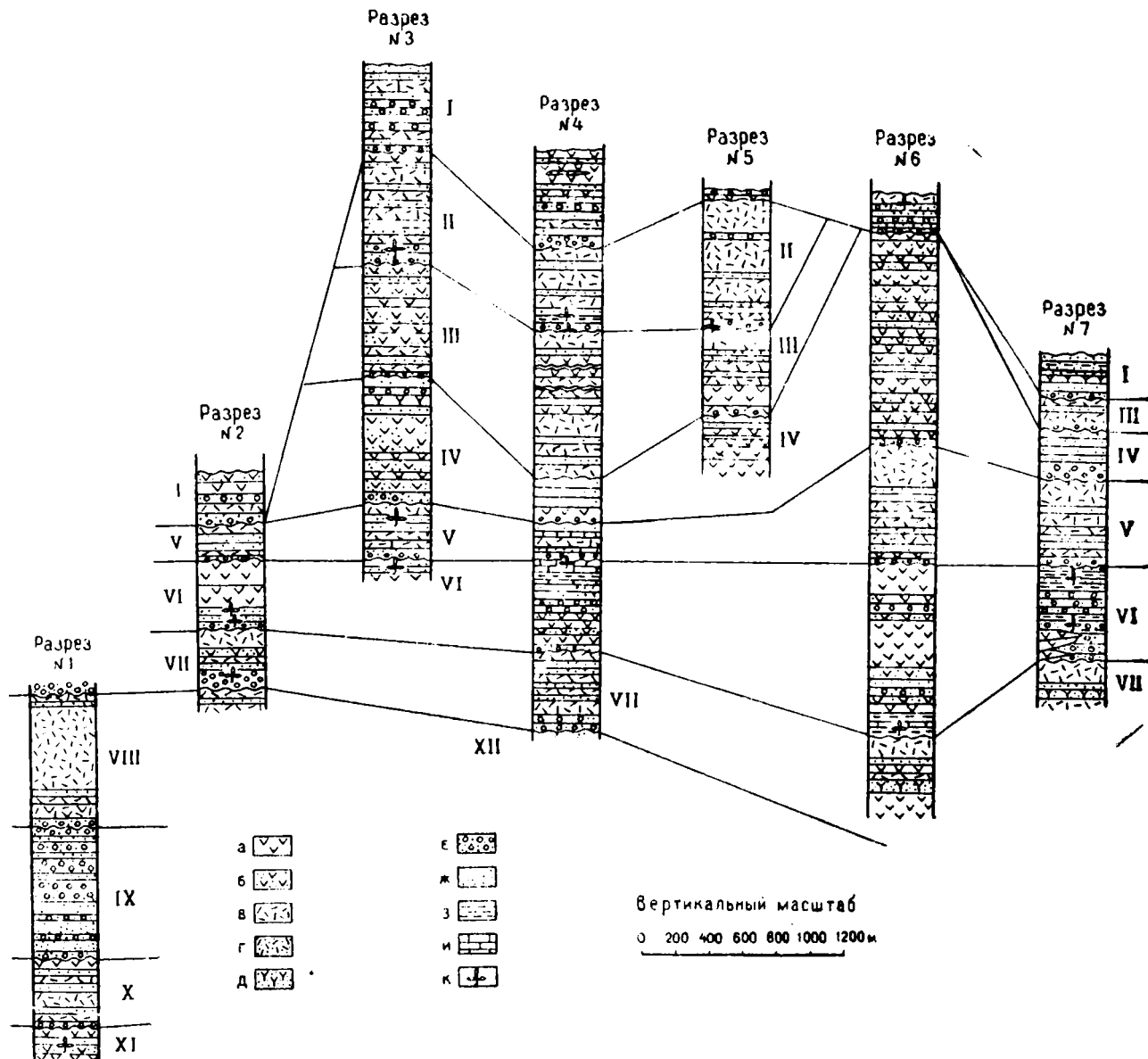
Рис. II—2. Схема сопоставления опорных разрезов Южной Джунгарии.
