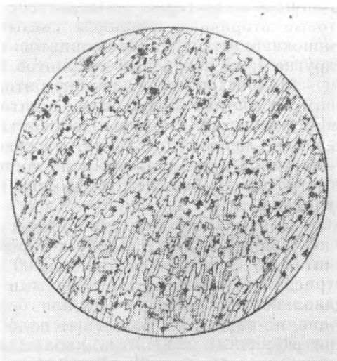
Рис. VI—6. Кварцево-каолинит-алунитовый вторичный кварцит. Ув. 110.
