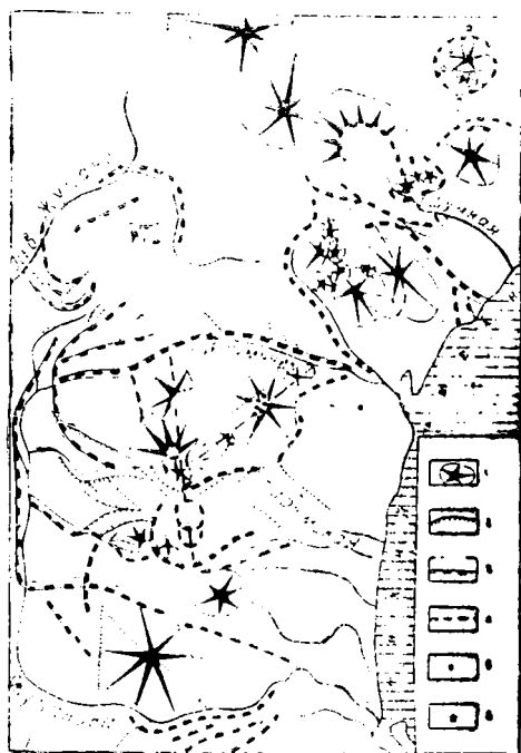
Рис. XVI—1. Кольцевые структуры и вулканы Карымско-Семьячинского района (по Э. Н. Эрлиху, 1966). 1 — вулканы, 2 — разломы, 3 — сбросы, ограничивающие вулcano-тектонические депрессии, 4 — предполагаемые разломы фундамента, контролирующие вулканические группы, 5 — кратеры, 6 — шлаковые конусы
