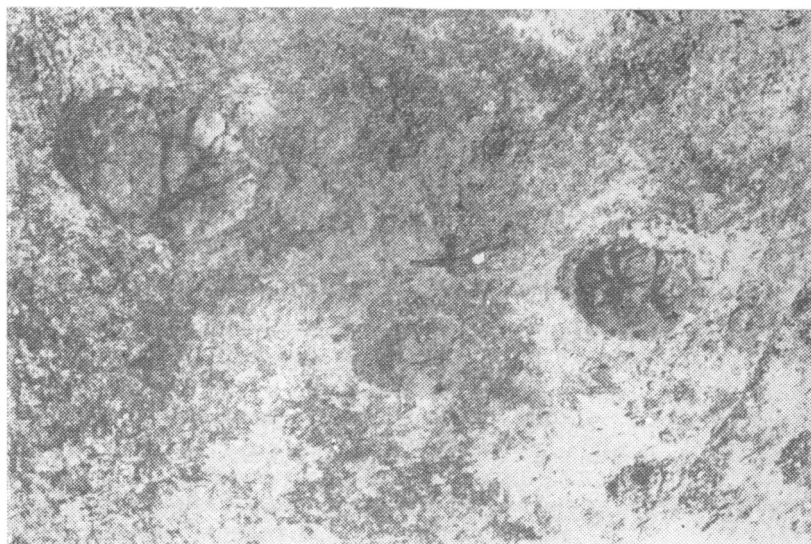
Рис. IV—30. Отпрепарированные андезитовые вулканические бомбы в составе конуроленской свиты. Горы Долантау.
