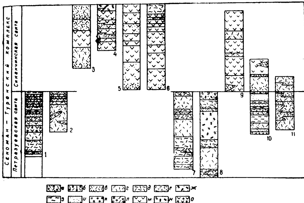
Рис. XI-3. Схема сопоставления разрезов сеноман-туронского комплекса. (а-г) — туфы кварцевых порфиров, липаритов, б — алгомеритовые, в — псефитовые, г — псаммитовые, д — игнимбиты, е — туфопесчаники, ж — туфы дацитов, з — алевролиты, и — песчаники, к — конгломераты, л — агломеративные туфы андезитов, м — андезиты, н — дациты, о — брекчиевые лавы андезитов.
