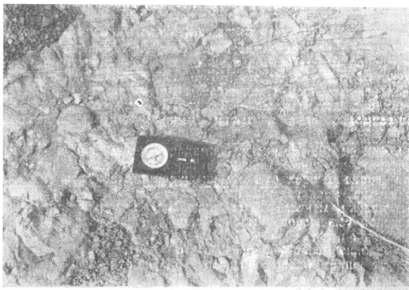
Рис. III—28. Лавобрекчии андезитов вокруг андезитовой экструзии в горах Архарлы
