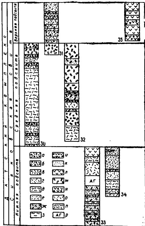
Рис. XI—5. Схема сопоставления разрезов датского комплекса.
