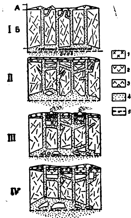
Рис. XIV—1. Схема развития вулканизма Восточно-Сихотэ-Алиньского пояса.
