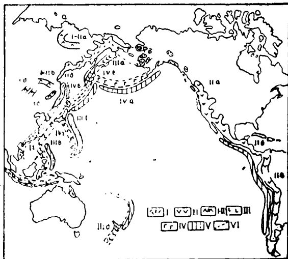
Рис. XVIII—1. Схема размещения вулканогенных поясов и зон Тихоокеанского кольца (по Ициско-ну, и др., 1965).
