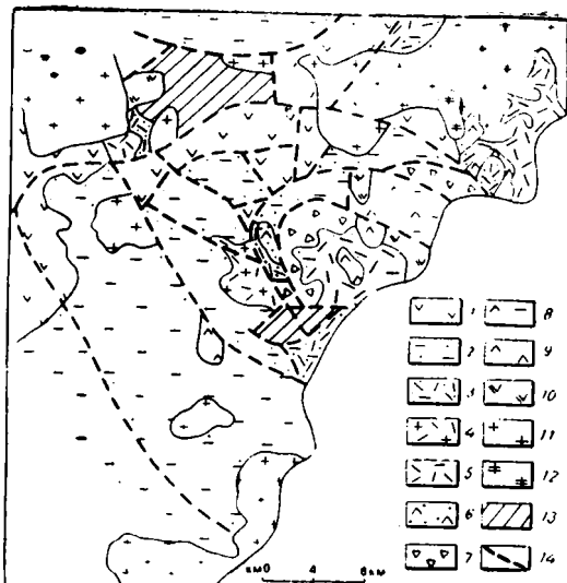
Рис. XII—2. Пластунская вулканотектоническая структура.
