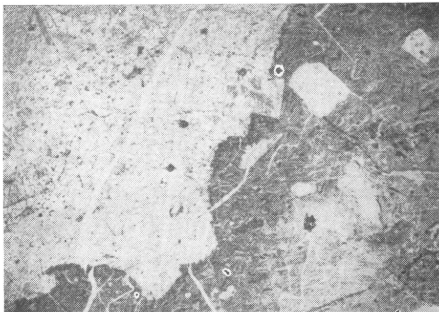
Рис. IV—13. Игнимбрит айнабулакского типа. Контакт шара (темное) и цементирующей массы. Вкрапленник плагиоклаза пересекает линию контакта. Ув. 60, при одном николе.
