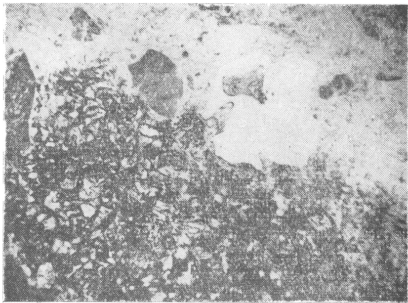
Рис. IV—3. Литоидный игнимбрит чебулайбулакского типа. Оплавленные обломки кварца и калишпата в сваренной пепловой массе. Ув. 60, при одном николе
