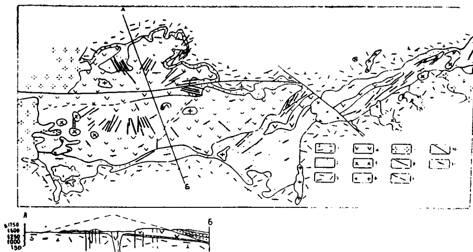
Рис. III—9. Схема геологического строения Конуроленского вулкана.
