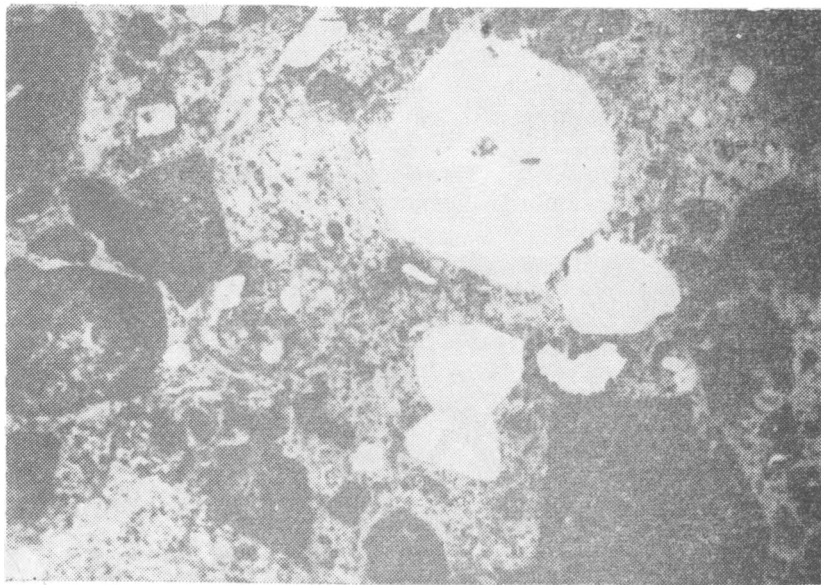
Рис. IV—32. Липарит. Вкрапленники калишпата и кварца в основной фельзитовой массе. Ув. 22, при одном никеле
