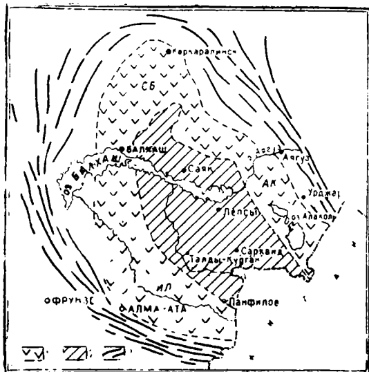
Рис. 1—1. Схема распространения верхнепалеозойских вулканогенных отложений.
