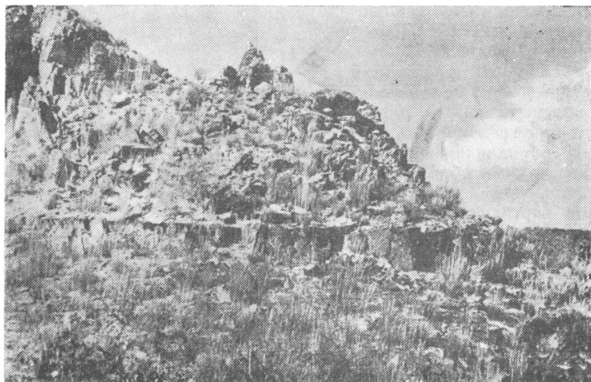
Рис. III—5. Силл кварцевых липаритов. Наблюдается четкий контакт с нижележащими туффитами. Горы Катутау.
