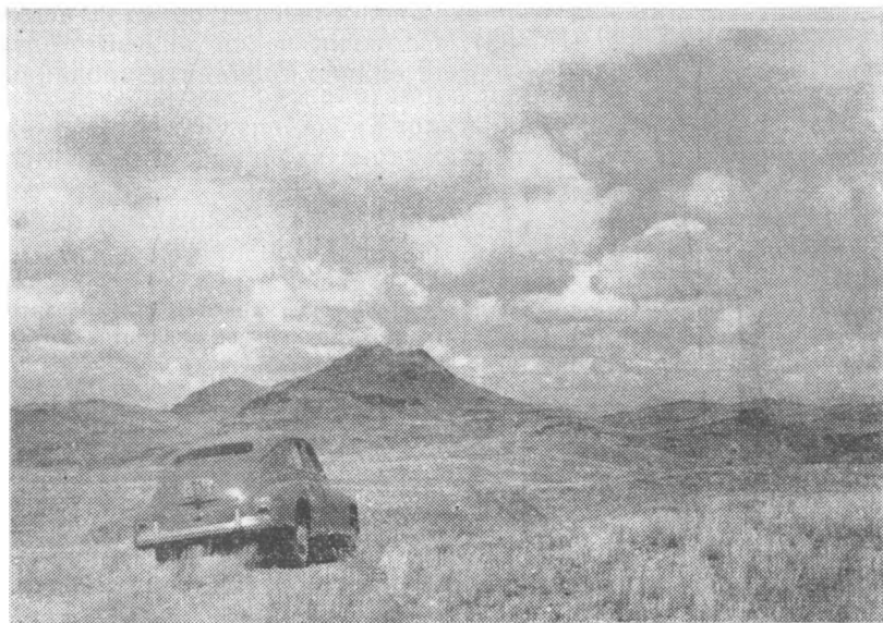
Рис. III—22. Андезитовый некк Майский в горах Катутау
