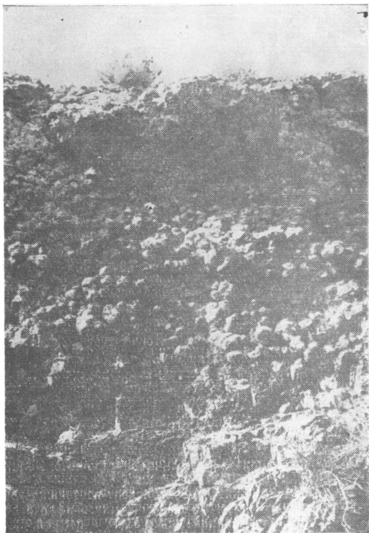
Рис. IV—7. Выход шаровых игнимбритов. Восточная часть гор Катутау.
