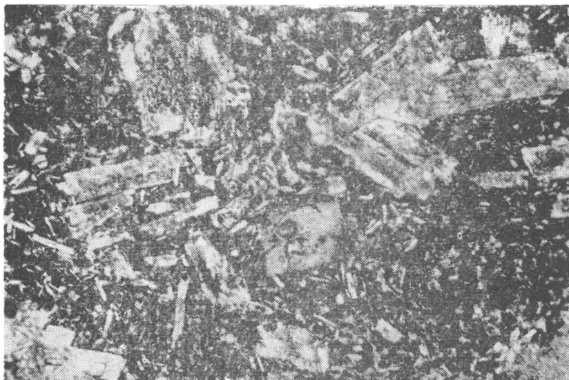
Рис. IV—26. Плагноклазовый андезит с серийно-порфировой структурой. Ув. 22, при скрещенных николях.
