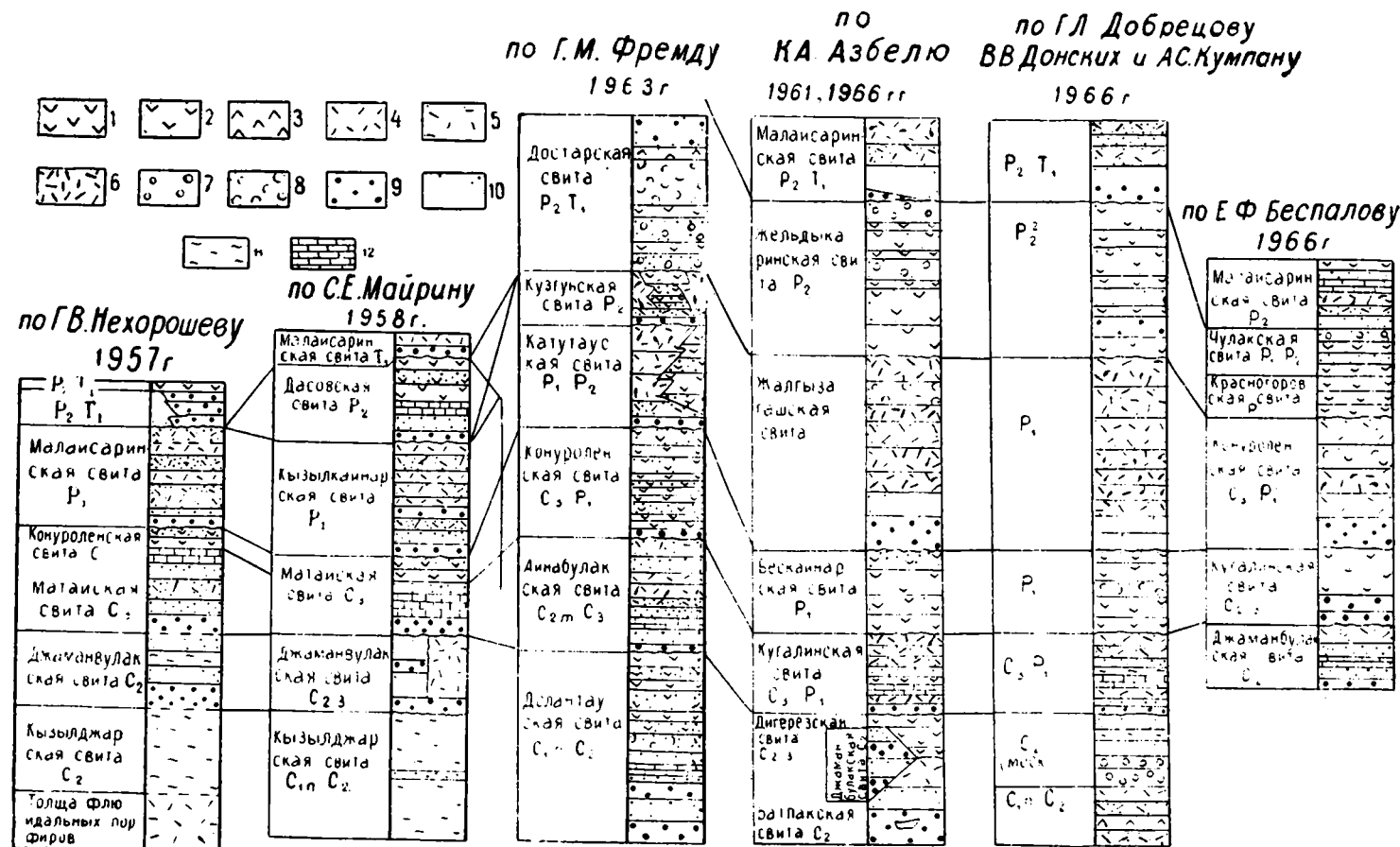
Рис. 1—3. Сопоставление стратиграфических схем верхнего палеозоя Джунгарского Алатау (по К. А. Азбелю, 1969)
