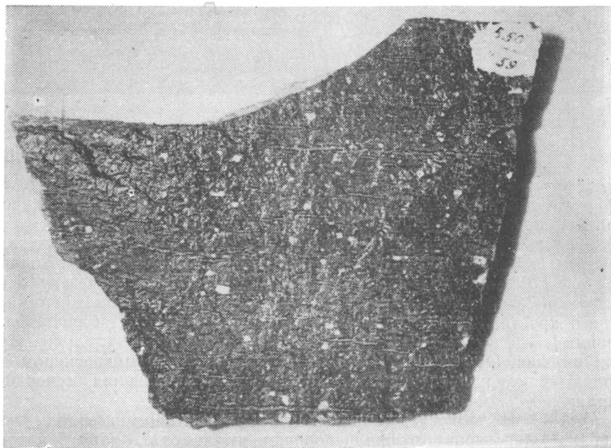
Рис. IV—15. Литондный игниспумит достарского типа. Параллельное расположение фьямме. \frac{2}{3} натур. величины.
