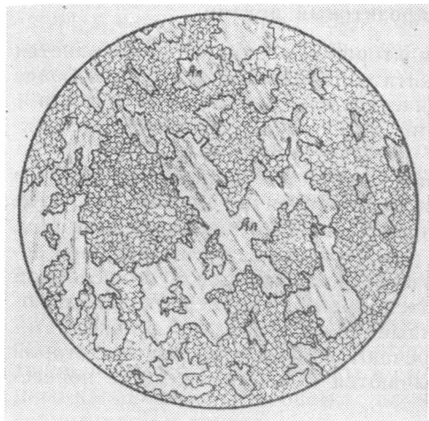
Рис. VI—7. Кварцево-алунитовый вторичный кварцит. Ув. 110.
