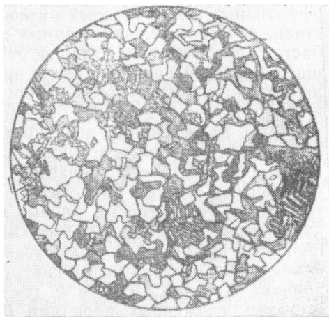
Рис. XIII — 11. Лейнократовый гранит. Приморская интрузивная серия. Ув. 22. Николит скрещены.
