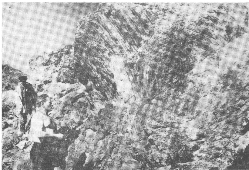
Рис. III—15. Койбинский вулкан. Экструзивные фельзиты с веерообразной флюиальностью.
