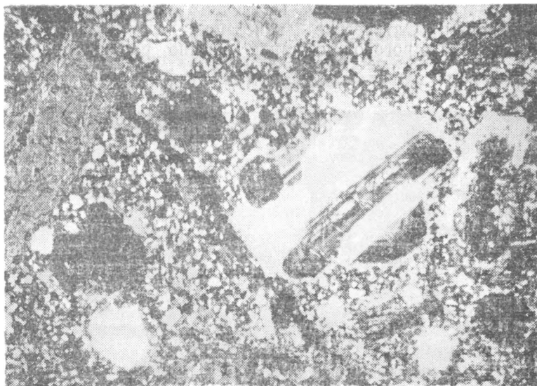
Рис. IV—48. Микрогранит-порфир. В микрогранулитовой основной массе вкрапленники зонального плагиоклаза, калишпата, биотита. Ув. 22, при скрещенных николях.
