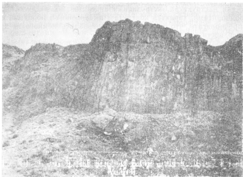
Рис. III—24. Андезито-базальтовый некк Арчуокский в горах Долантау
