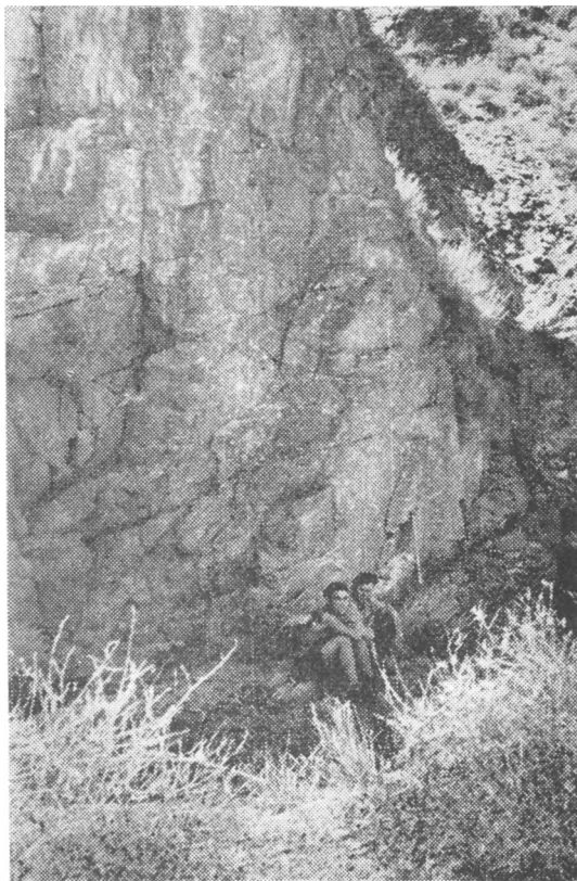
Рис. IV—18. Выходы игниспумитов еккульского типа. Лог Еккуль.
