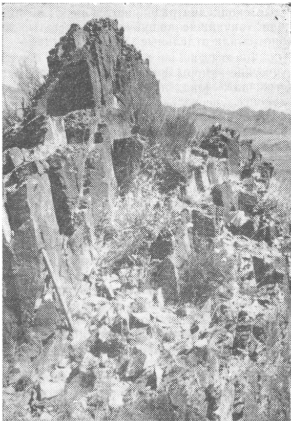
Рис. III—16. Столбчатая отдельность в экструзивных фельзитах. Горы Катутау.
