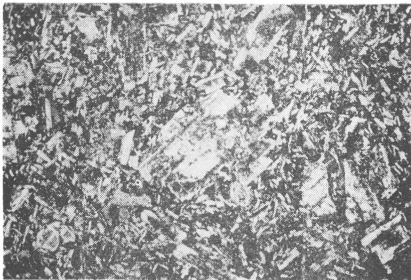
Рис. IV—25. Плагноклазовый андезит с интерсертальной структурой основной массы. Ув. 22, при скрещенных николях.
