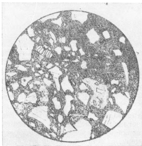
Рис. XIII — 5. Липаритовый игниспумит. Приморская свита. Ув. 22, при одном никеле
