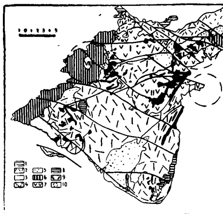
Рис. III—6. Схема размещения верхнепалеозойских андезитовых стратовулканов в г. Катутау.
