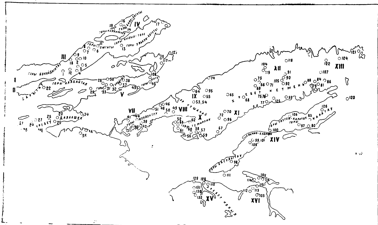
Рис. VII — 1. Схема расположения опорных разрезов Северного Тянь-Шаня
