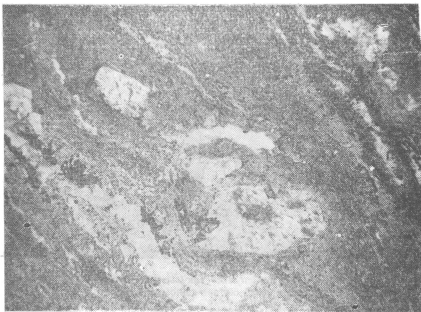
Рис. IV—20. Литонидный игниспумит ескульского типа. Флюидальне-полосчатая структура основной массы. Ув. 22, при одном никеле.
