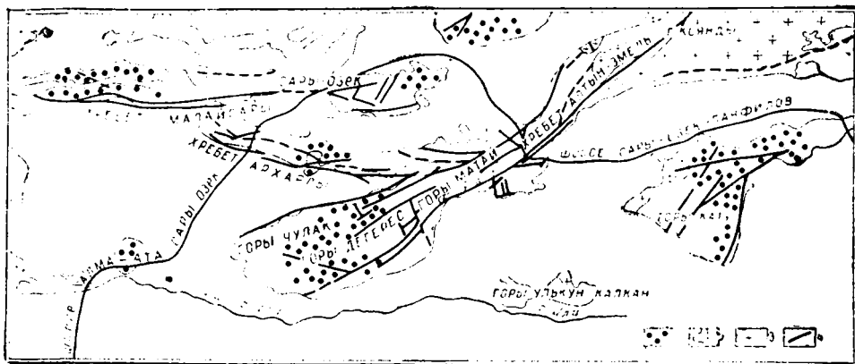
Рис. VI—1. Схема размещения гидротермально измененных пород Южной Джунгарии.
