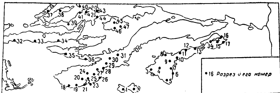
Рис. II—3. Схема расположения разрезов Южной Джунгарии
