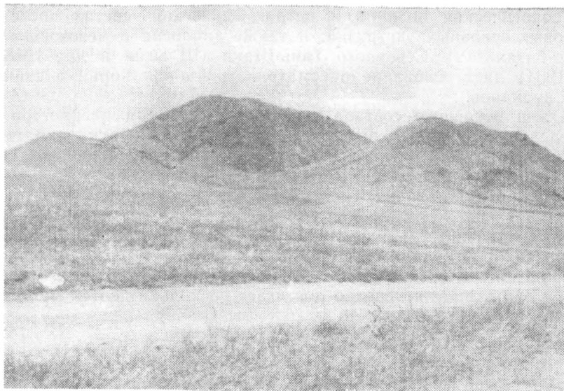
Рис. III—25. Фельзитовый некк Кызылчеку в горах Архарлы
