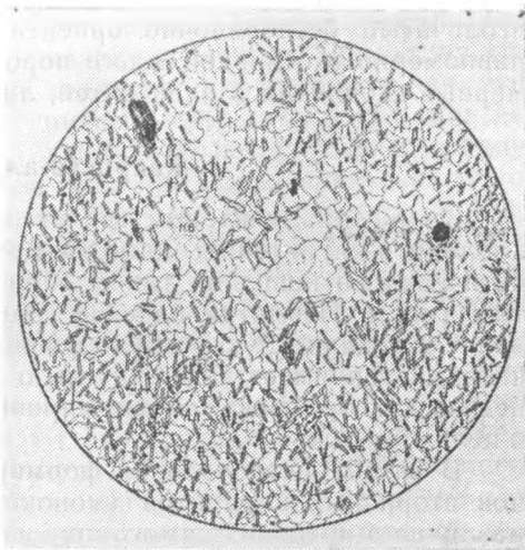
Рис. VI—5. Кварцево-каолинит-алунитовый вторичный кварцит. Ув. 110.
