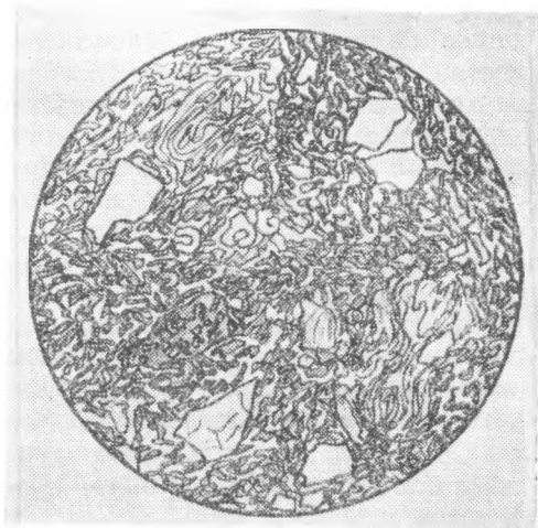
Рис. XIII—3. Липарито-дацитовый игнимбрит с пепловой структурой основной массы. Обломки зерен кварца обтекаются пепловыми частицами. Приморская свита. Ув. 22, при одном николе
