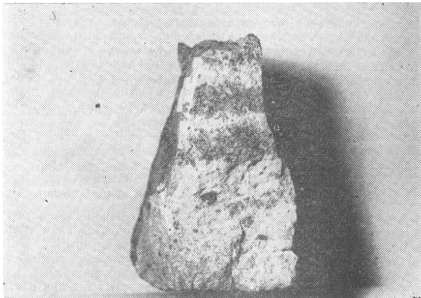
Рис. IV—23. Литоидный игниспумит ташкумырсайского типа. 3/4 натур. величины.
