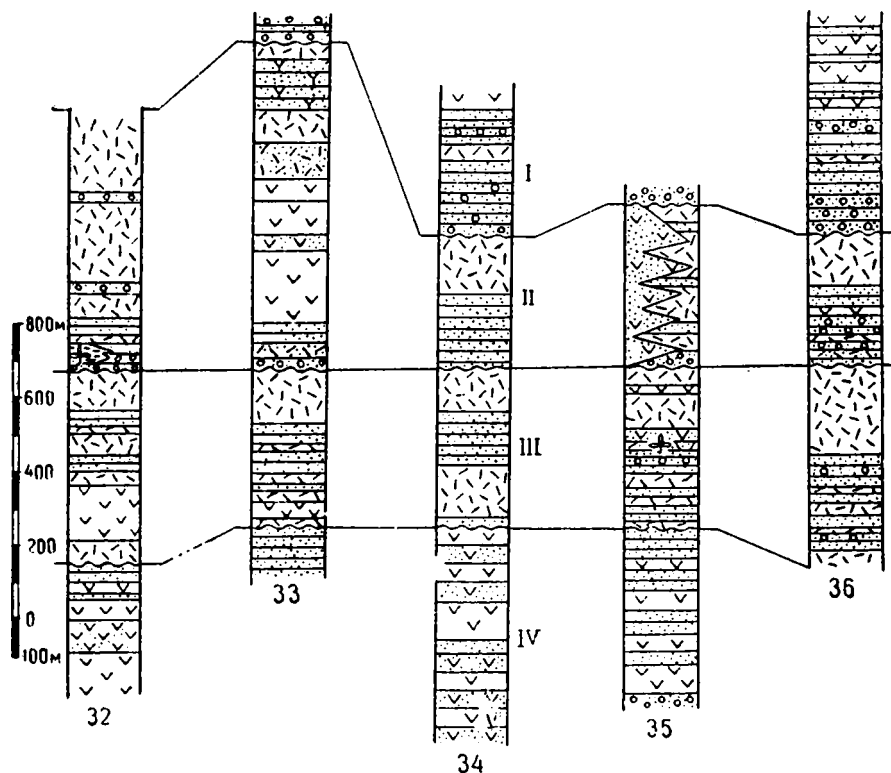
Рис. II—6. Схема сопоставления разрезов Южной Джунгарии. (Условные обозначения на рис. II—2).
