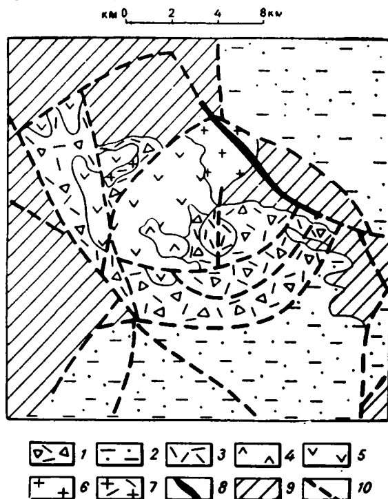
Рис. XII—5. Солонцовская вулcano-тектоническая структура.
