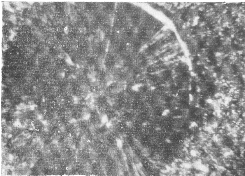
Рис. IV—12. Игнимбрит айнабулакского типа. Радиально-лучистое строение микрошара. Ув. 60, при скрещенных николях.
