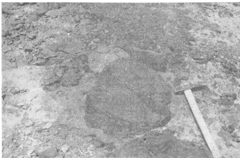
Рис. IV—40. Лахаровые брекчий в долантауской свите. Горы Долантау.
