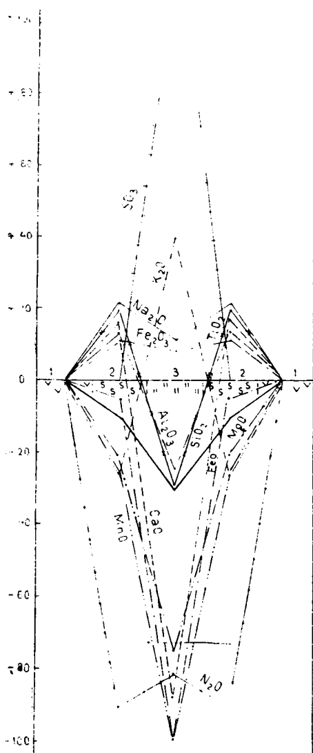
Рис. VI—8. Вариационная диаграмма «привнос — вынос» при метасоматической зональности ащибастауского типа (к табл. VI—1).
