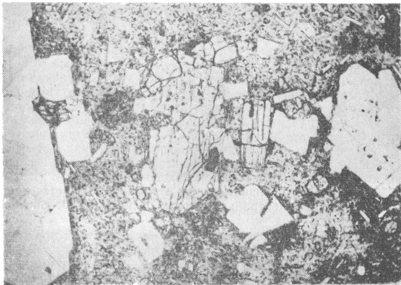
Рис. IV—27. Плагиоклаз-пироксеновый андезит. Крупные вкрапленники плагиоклаза и пироксена в основной массе с гналопиллитовой структурой. Ув. 22, при одном никеле.
