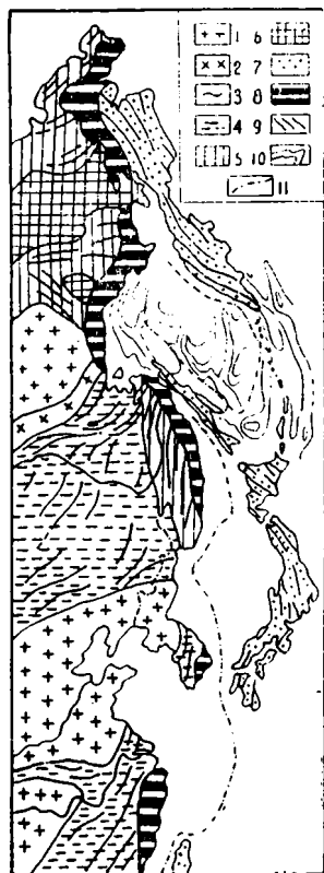
Рис. XVIII — 5. Схема структурного положения Восточно-Азиатского вулканического пояса (по М. С. Нагибиной, 1964):
