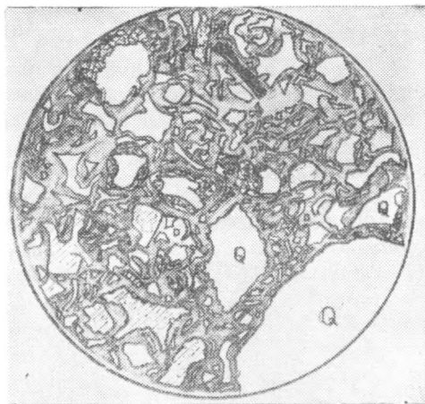
Рис. XIII—4. Слабо сваренный липаритовый игнимбрит с пепловой структурой основной массы. Приморская свита. Ув. 22, при одном никеле
