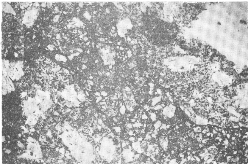
Рис. IV—42. Витрокристаллокластический туф. Ув. 22, при одном никеле.
