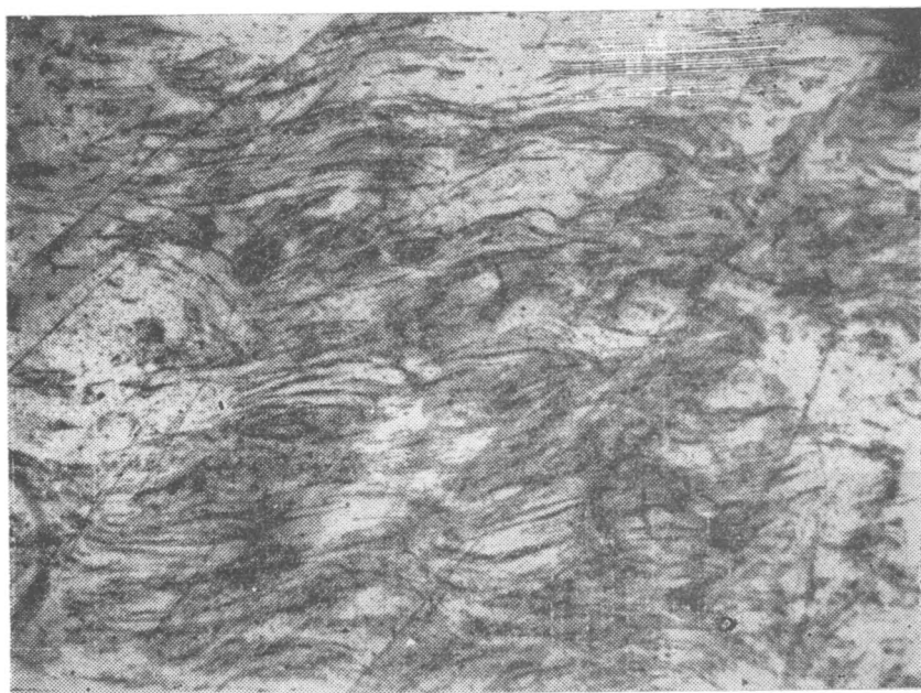
Рис. IV—34. Вулканическое стекло с флюктуационной текстурой. Ув. 60, при одном никеле.
