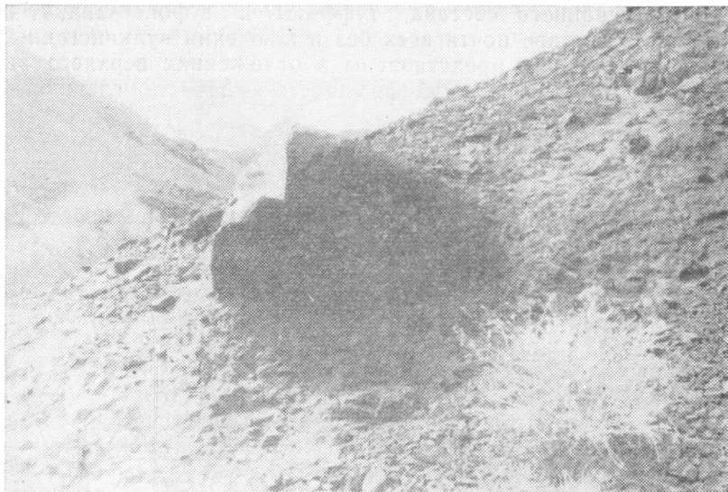
Рис. IV—39. Лахаровые брекчий в достарской свите. Горы Катутау.
