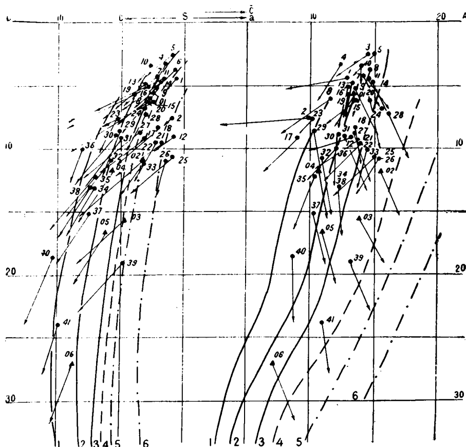
Рис. V—7. Петрохимическая диаграмма постпермских интрузивных пород.
