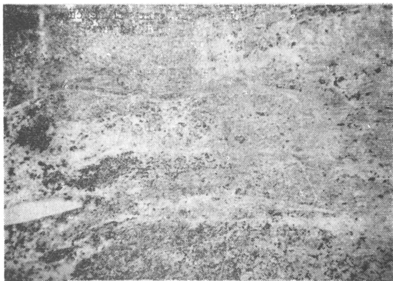
Рис. IV—24. Литоидный игниспумит ташкумырсайского типа. Флюидально-полосчатое строение. Ув. 22, при одном никеле.
