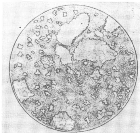
Рис. XIII—7. Фельзит с пятнистой текстурой. Приморская свита. Ув. 22, при одном никеле
