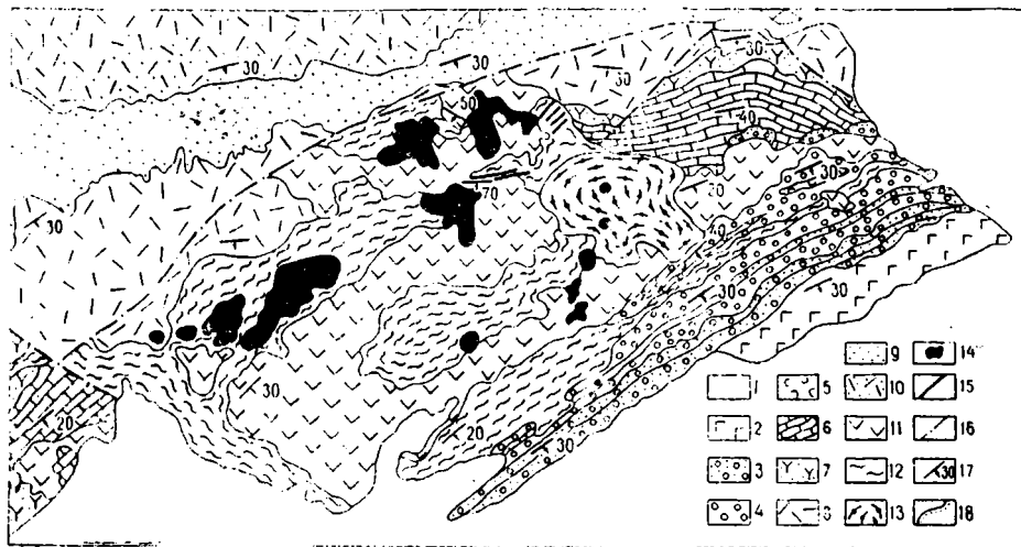
Рис. III—14. Схема геологического строения Койбинского вулкана.
