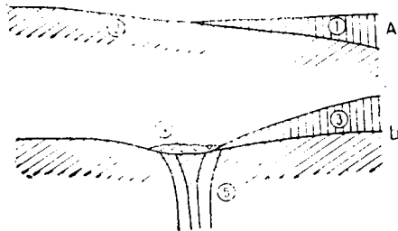
Рис. 1—2. Схема развития Джунгарского верхнепалеозойского компенсационного прогиба.
