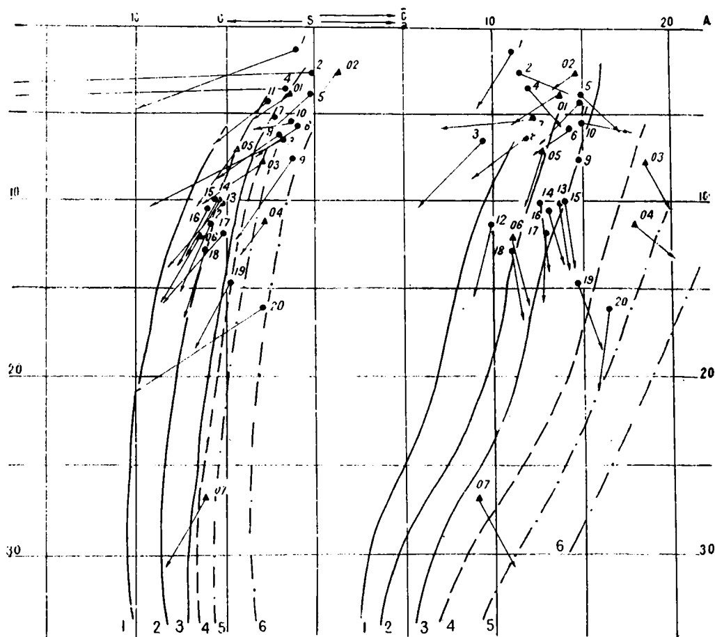
Рис. V—5. Петрохимическая диаграмма постпермских экструзивных пород.
