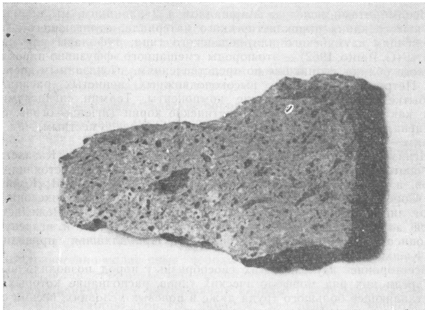
Рис. IV—1. Литоидный игнимбрит чебулайбулакского типа. Субпараллельное, кулисообразное расположение фьямме. Натур. величина.
