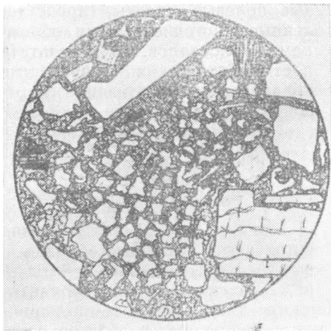
Рис. XIII—1. Сильно сваренный липаритовый игнимбрит с фельзитовой структурой основной массы. Приморская свита. Ув. 22, при одном никеле.
