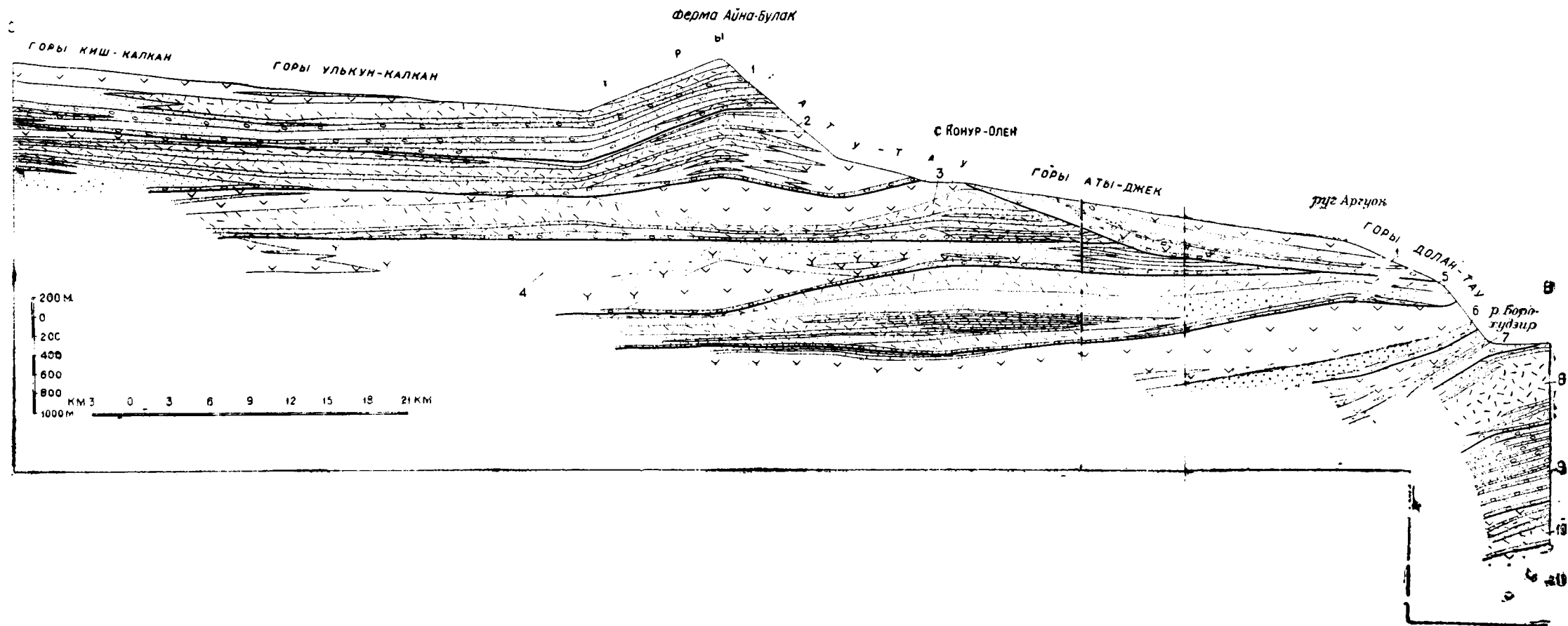
Рис. 11—9. Схема фациальной изменчивости средне-верхнепалеозойских вулканогенных свит Южной Джунгарии. Восточная часть региона. 1 — достарская свита; 2 — кузгунская свита; 3 — катутауская свита; 4 — конуроленская свита; 5 — айнабулакская свита; 6 — долантауская свита; 7 — куарасанская свита; 8 — борохудзирская свита; 9 — коктаасская свита; 10 — дуваптауская свита; 11 — алтынэмельская свита. (Условные обозначения на рис. 11—2).
