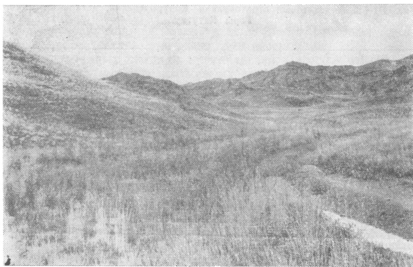
Рис. III—7. Андезитовый стратовулкан Конуроленский. Общий вид. Горы Катутау.
