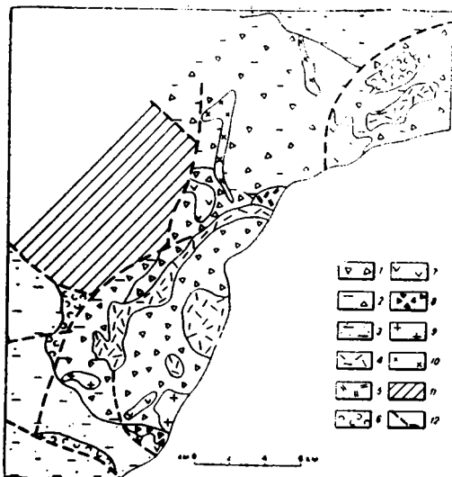
Рис. XII—4. Бринеровская вулcano-тектоническая структура.
