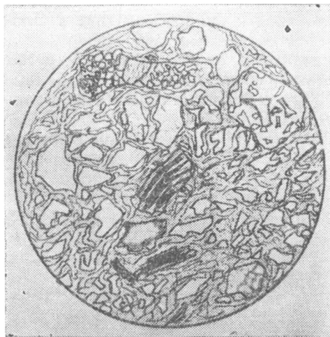
Рис. XIII—2. Липаритовый игнимбрит с чешуйками биотита. Основная масса сильно сварена. Сияновская свита. Ув. 22, при одном николе
