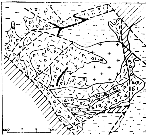
Рис. XII—3. Тетюхинская вулcano-тектоническая структура.
