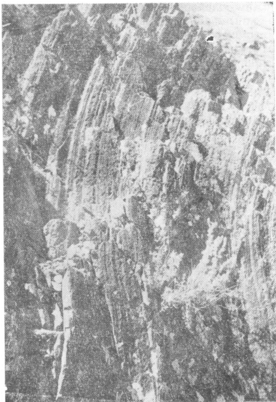
Рис. III—4. Вертикальная отдельность в экструзивных фельзитах, развивающаяся по флюидалности. Горы Катутау.
