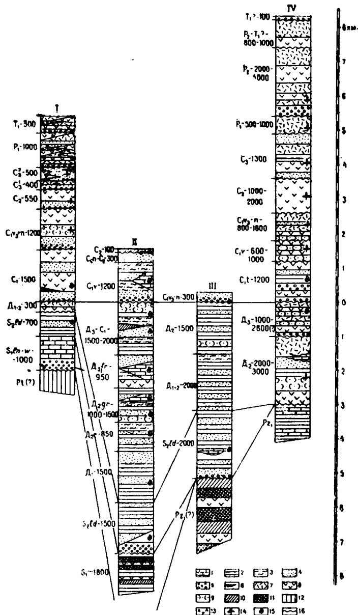
Рис. 1—4. Схема сопоставления разрезов структурно-фациальных зон. I — Илийская зона, II — Таставская зона, III — Кентерлау-Саркандская зона. IV — Токрау-Алаккульская зона.
