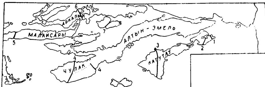
Рис. II—1. Схема расположения опорных разрезов Южной Джунгарии
