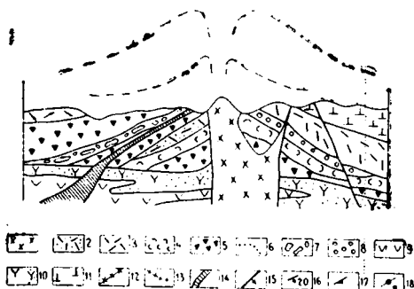
Рис. III—3. Схема геологического строения Кожамджарского вулкана.
