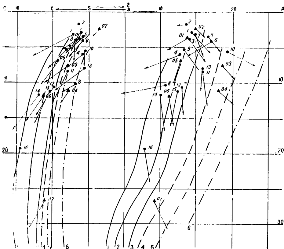
Рис. V—1. Петрохимическая диаграмма каменноугольных эффузивных пород.
