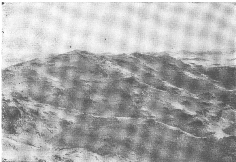
Рис. III—8. Андезитовый стратовулкан Конуроленский, деталь строения. Горы Катутау.
