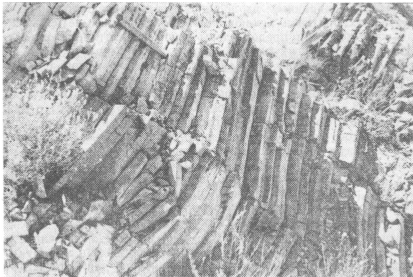
Рис. III—19. Тонкостолбчатая отдельность в экструзивных фельзитах. Горы Катутау.
