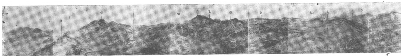
Рис. III—2. Общий вид Кожамджарского вулкана. ф — фельзиты Центрального нека; и — игниспумиты; а — агломераты; л — лахары; ан — андезитовый силл
