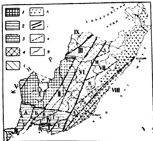
Рис. X-3. Схема геолого-структурного районирования Приморского края (по И. И. Берсеневу, 1968).
