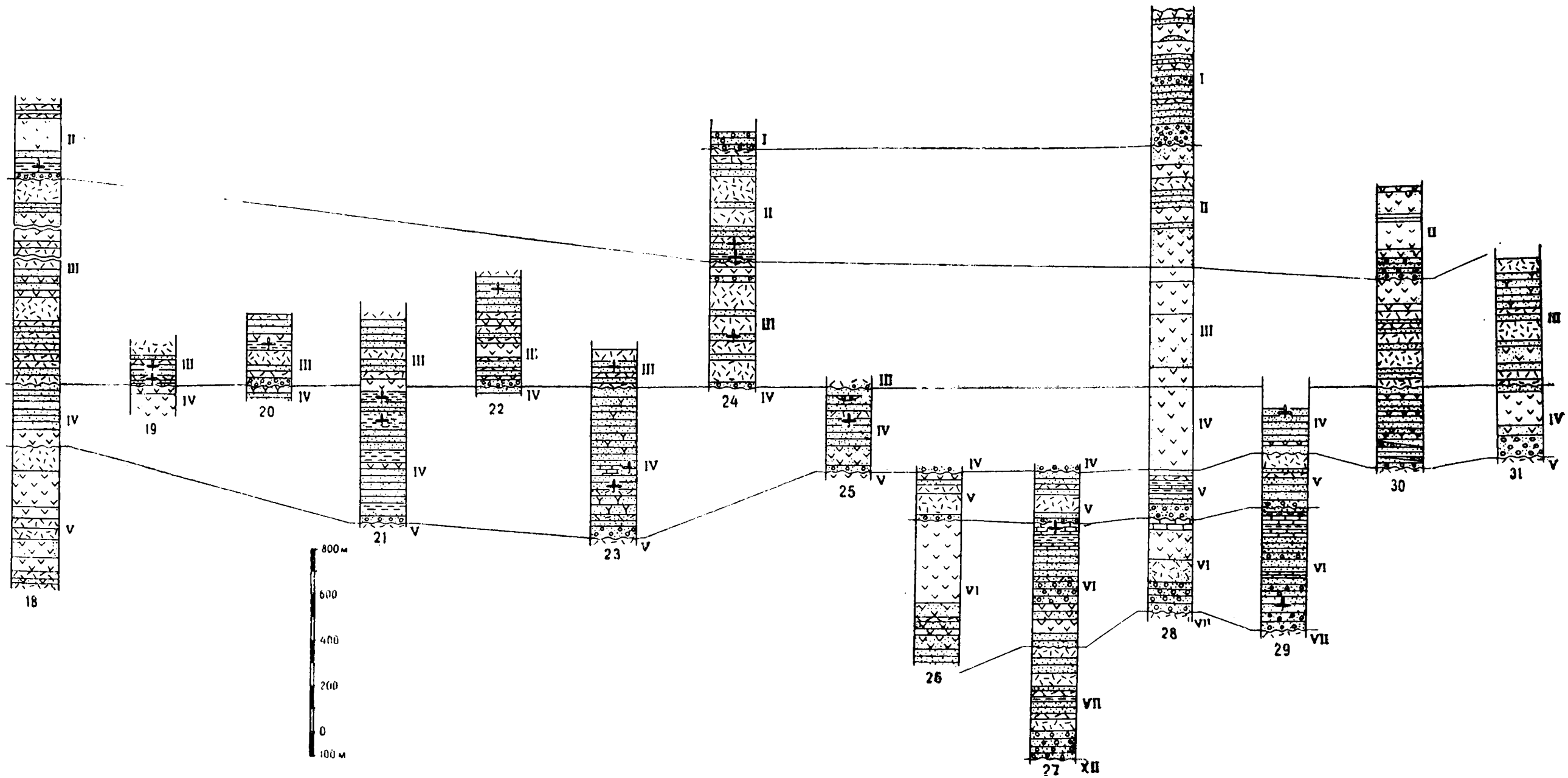
Рис. II—5. Схема сопоставления разрезов Южной Джунгарии. (Условные обозначения на рис. II—1).
