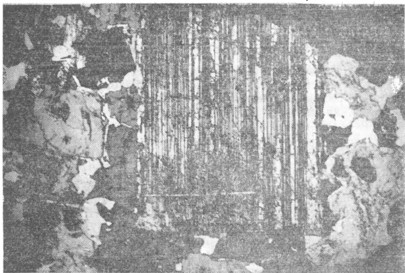
Рис. IV—46. Кварцевый монзонит-порфир. Вкрапленник лабрадора в основной массе с монзонитовой структурой. Ув. 22, при скрещенных николях.
