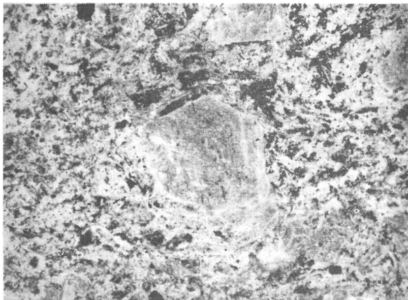
Рис. IV—2. Литоидный игнимбрит чебулайбулакского типа. Сваренная пепловая масса обтекает обломок калишпата. Ув. 40, при одном никеле.
