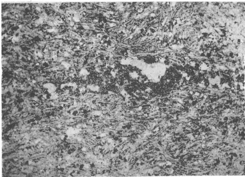
Рис. IV—29. Андезито-базальт с пилотакситовой и гналопилитовой структурой основной массы. Ув. 22, при одном никеле.
