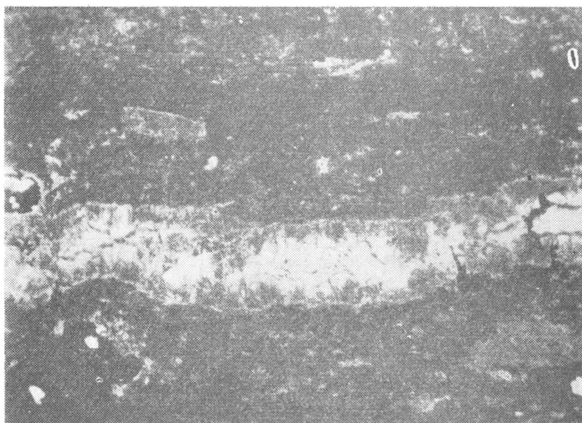
Рис. IV—17. Литоидный игниспумит достарского типа. Деталь строения линзочки. Ув. 110, при одном николе.
