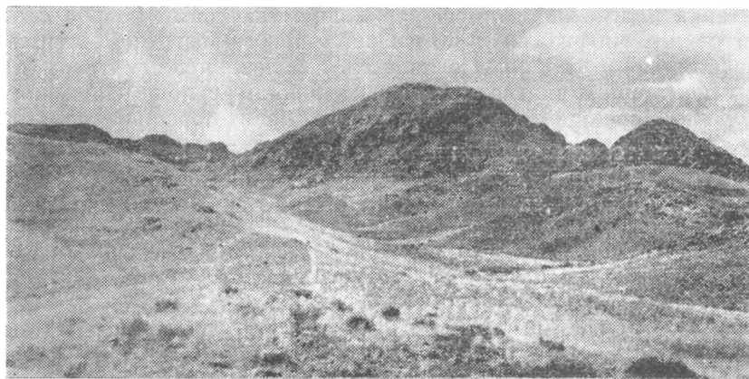
Рис. III—21. Фельзитовый некк Июльский. Горы Катутау
