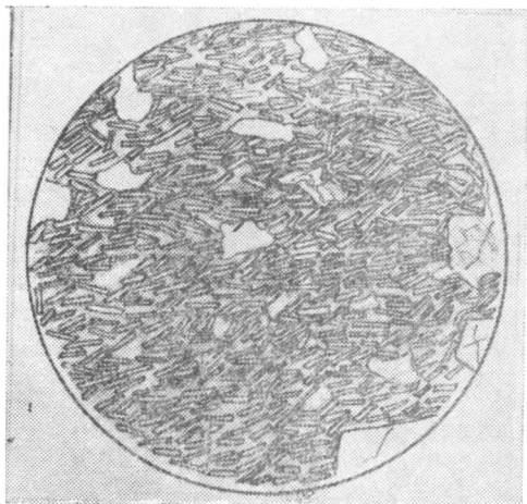
Рис. XIII—6. Плагиоклазовый андезит. Сияновская свита. Ув. 22, при одном николе
