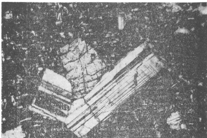
Рис. IV—37. Авгит-гиперстеновый андезито-базальт. Ув. 60, при скрещенных николях
