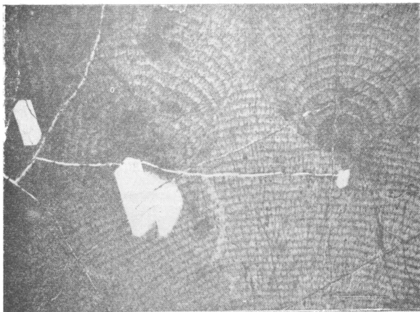
Рис. IV—35. Концентрически зональное строение шаровых обособлений в вулканическом стекле. Ув. 22, при одном николе.
