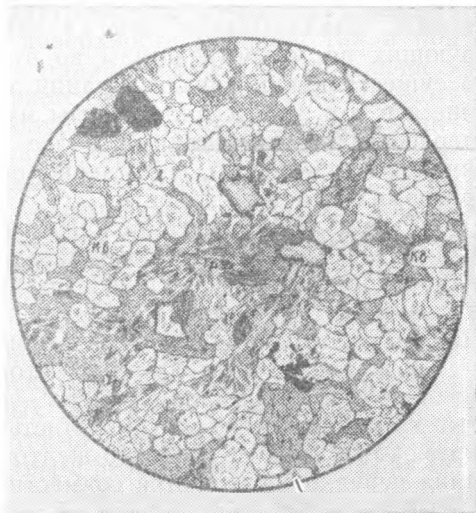
Рис. VI—2. Кварцево-мусковитовый вторичный кварцит. Ув. 110
