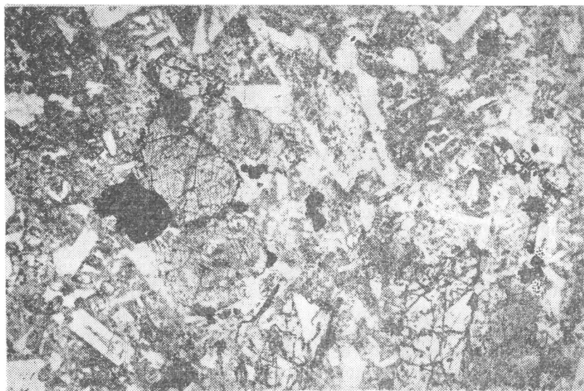
Рис. IV—45. Кварцевый монзонит. Резкий идиоморфизм плагиоклаза по отношению к калишпату (монзонитовая структура). Ув. 22, при одном николе.
