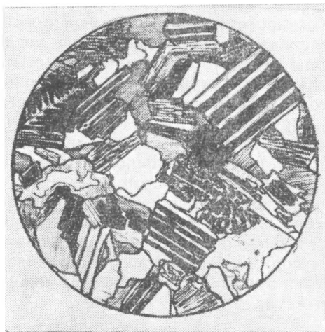
Рис. XIII — 10. Кварцевый диорит. Приморская интрузивная серия. Ув. 22, при скрещенных николях.
