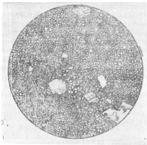
Рис. XIII—12. Алунино-каолинитовый вторичный кварцит по туфам кислого состава. Ув. 22. Николи скрещеньи
