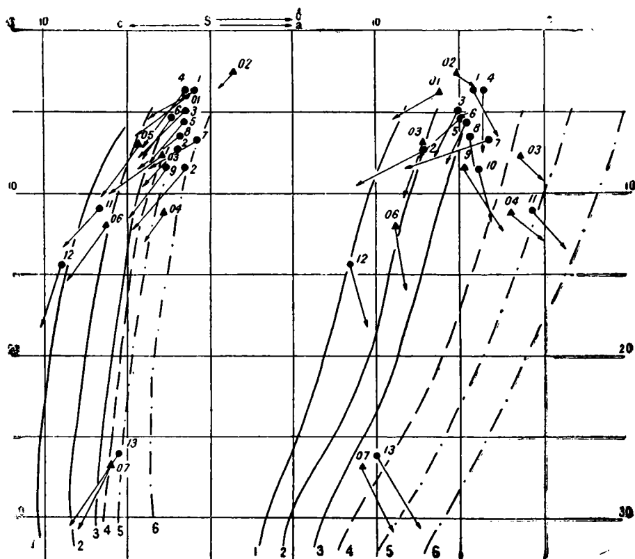
Рис. V—4. Петрохимическая диаграмма нижнетриасовых эффузивных пород.
