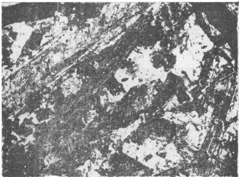
Рис. IV—38. Спессартит. Призматически-игольчатые кристаллы роговой обманки и плагиоклаза. Ув. 22, при скрещенных николях.
