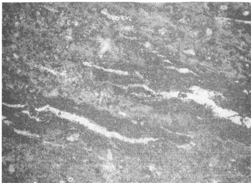
Рис. IV—16. Литоидный игниспумит достарского типа. Параллельное расположение линзочек (фьямме). Ув. 60, при одном николе.
