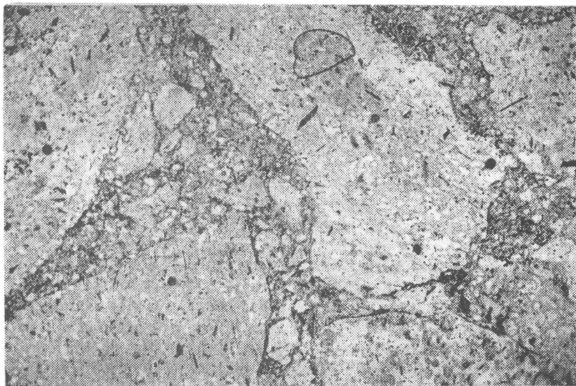
Рис. IV—41. Туфоагломерат. Обломки сцементированы туфовым материалом. Ув. 22, при одном никеле.
