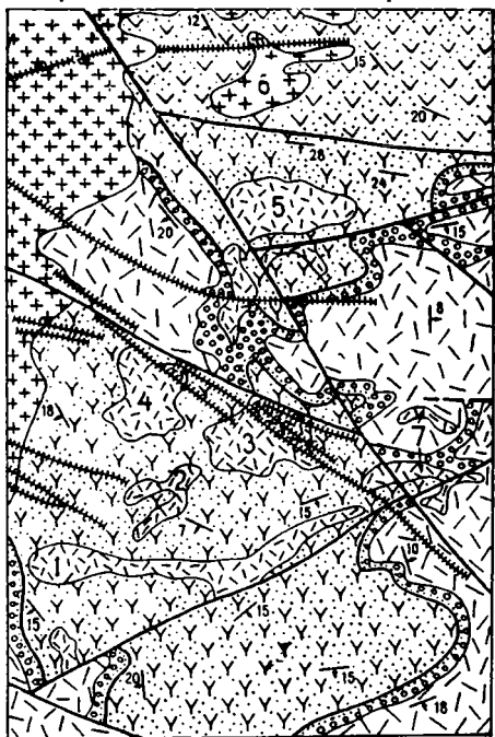
Рис. III—17. Схема геологического строения района Южной группы некков в горах Катутау.
