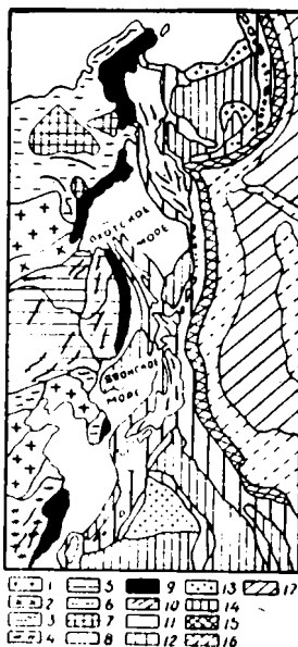
Рис. X—1. Структурное положение Восточно-Азиатского вулканического пояса. По тектонической карте Евразии, 1966. 1 — древние платформы, 2 — области протерозойской складчатости Станового хребта, 3 — области байкальской складчатости, 4 — области каледонской складчатости, 5 — области герцинской складчатости, 6 — области мезозойской складчатости, 7 — срединные массивы в области мезозойской складчатости, 8 — области камчатской складчатости, 9 — Восточно-Азиатский вулканический пояс, 10 — линии простиралий. Структуры морского и океанического дна: 11 — участки эоно-мезозойских и более древних платформ, 12 — кайнозойские складчатые и геосинклинальные области, 13 — участки донегеновой складчатости, 14 — глубокие котловины, лишенные гранитного слоя, 15 — глубоководные желоба, 16 — сводовые океанические поднятия, 17 — океанические плиты.
