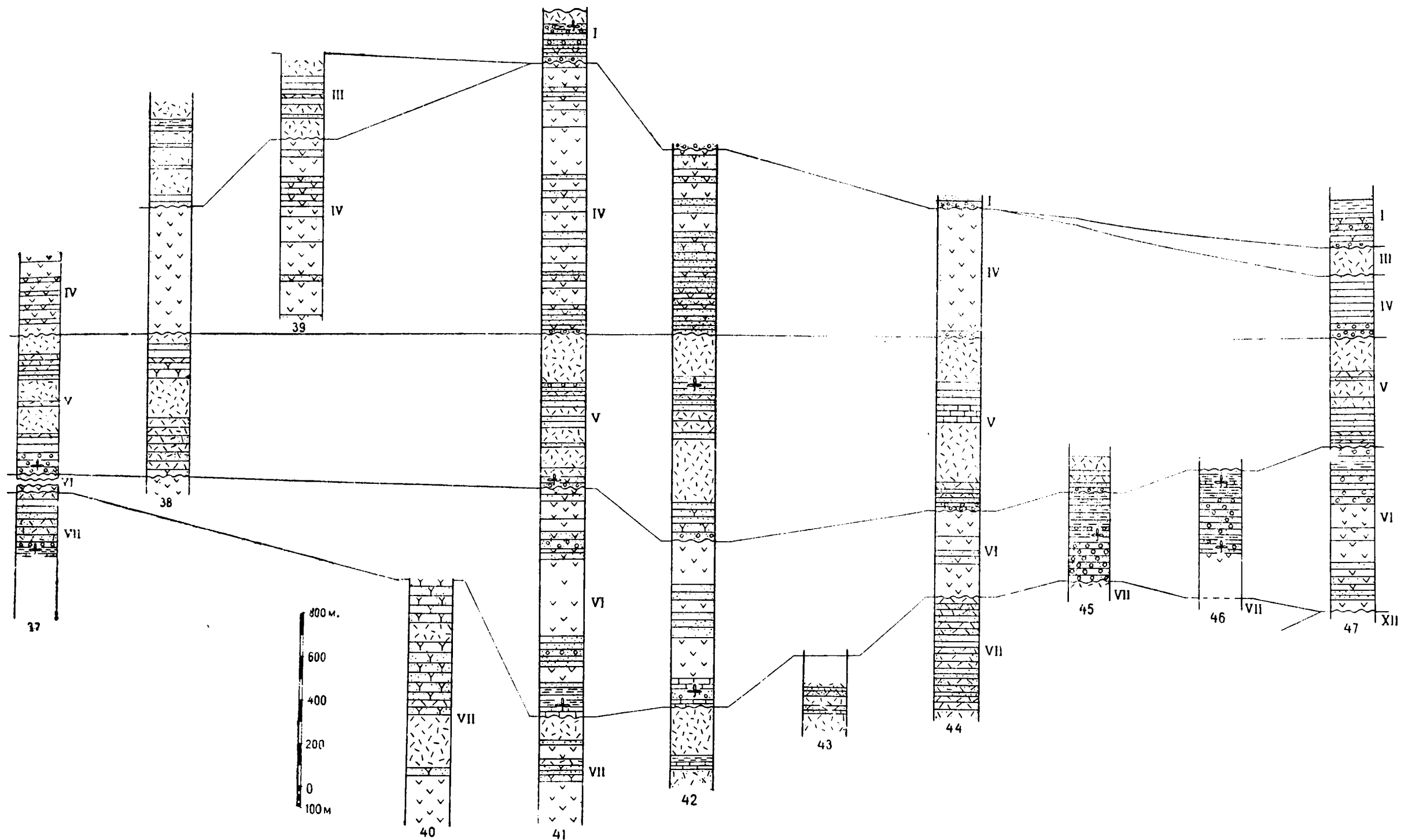
Рис. II—7. Схема сопоставления разрезов Южной Джунгарии. (Условные обозначения на рис. II—2).
