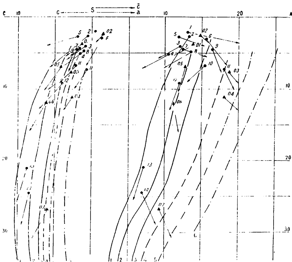
Рис. V—2. Петрохимическая диаграмма нижнепермских эффузивных пород.
