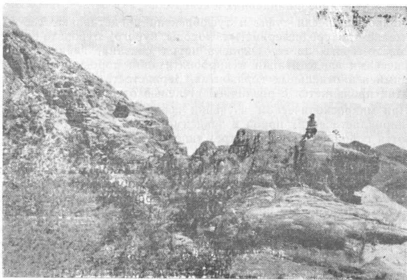
Рис. III—20. Дайка плагиосиенит-порфиров, рвущая фельзиты Южного некка. Горы Катутау
