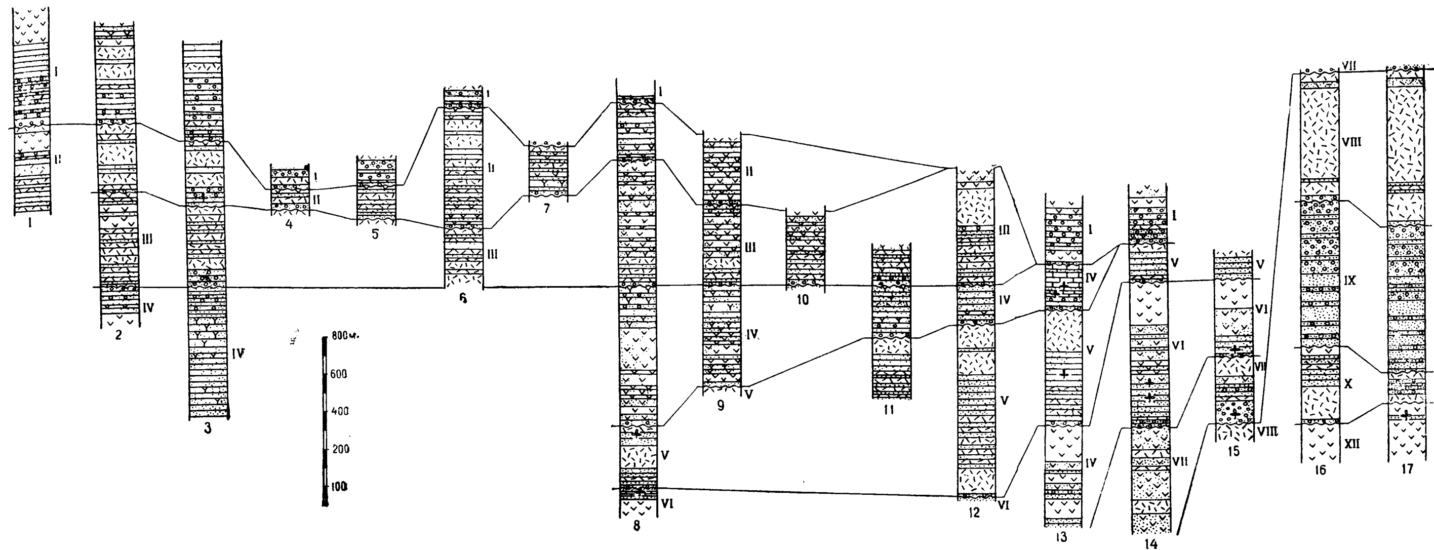
Рис. II—4. Схема сопоставления разрезов Южной Джунгарии. (Условные обозначения на рис. II—2).
