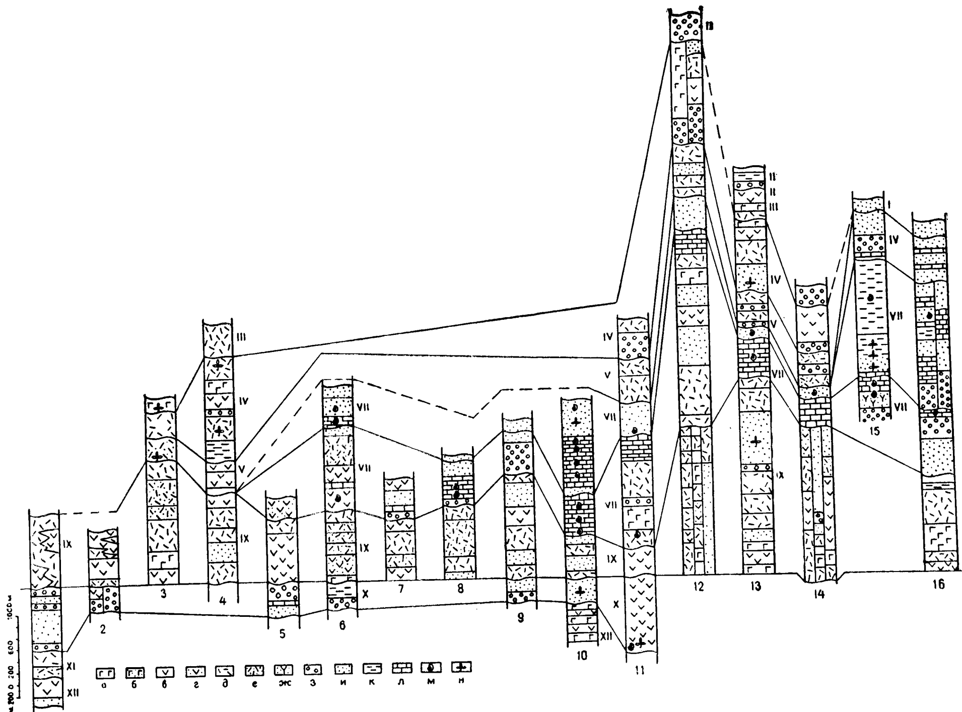
Рис. VII—2. Схема сопоставления разрезов Северного Тянь-Шаня (по материалам Б. П. Блинова, П. А. Сушкова, Н. М. Чабдарова и др.).
