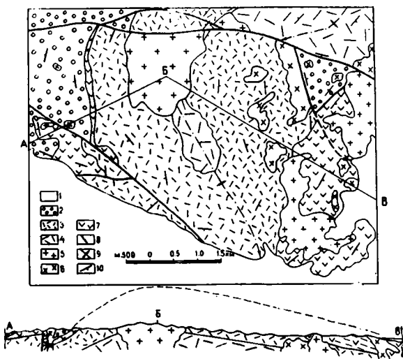
Рис. III—11. Схема геологического строения Ашибастауского стратовулкана.
