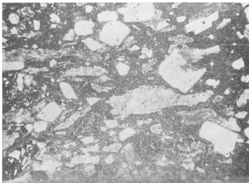
Рис. IV—5. Стекловатый игнимбрит архарлинского типа. Флюидальная текстура основной массы. Ув. 45, при одном николе.
