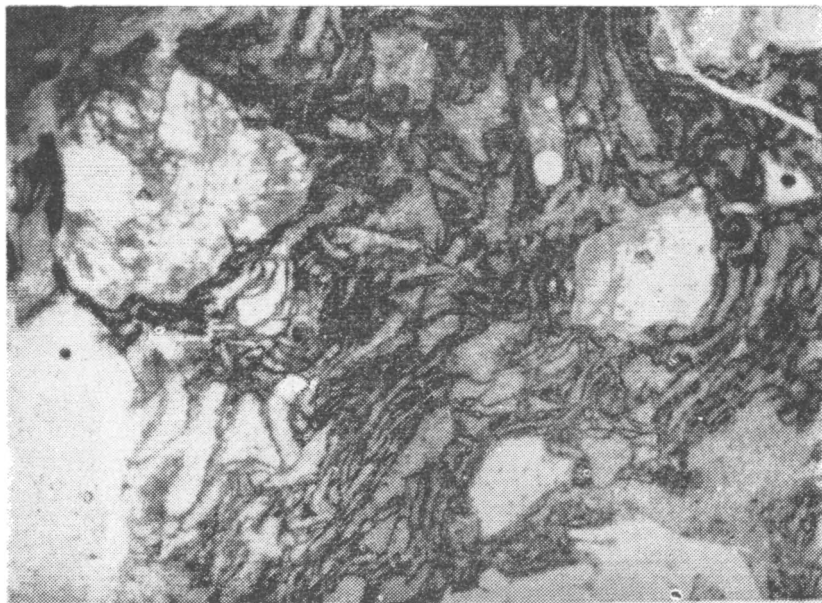
Рис. IV—8. Шаровой игнимбрит айнабулакского типа. Контуры пепловых частиц подчеркиваются оторочкой из мельчайших зерен гематита. Ув. 22. при одном николе
