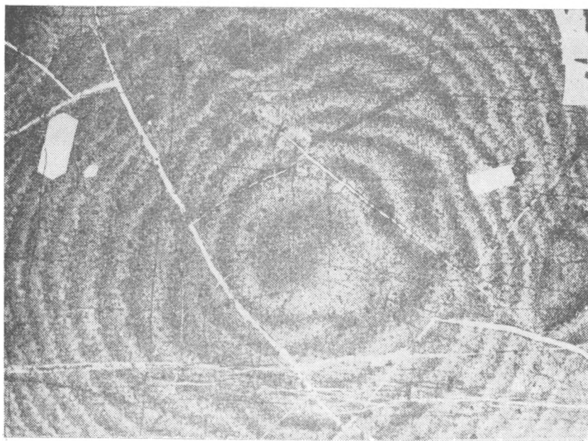
Рис. IV—36. Концентрически зональное строение шаровых обособлений в вулканическом стекле. Деталь строения. Ув. 60, при одном николе.
