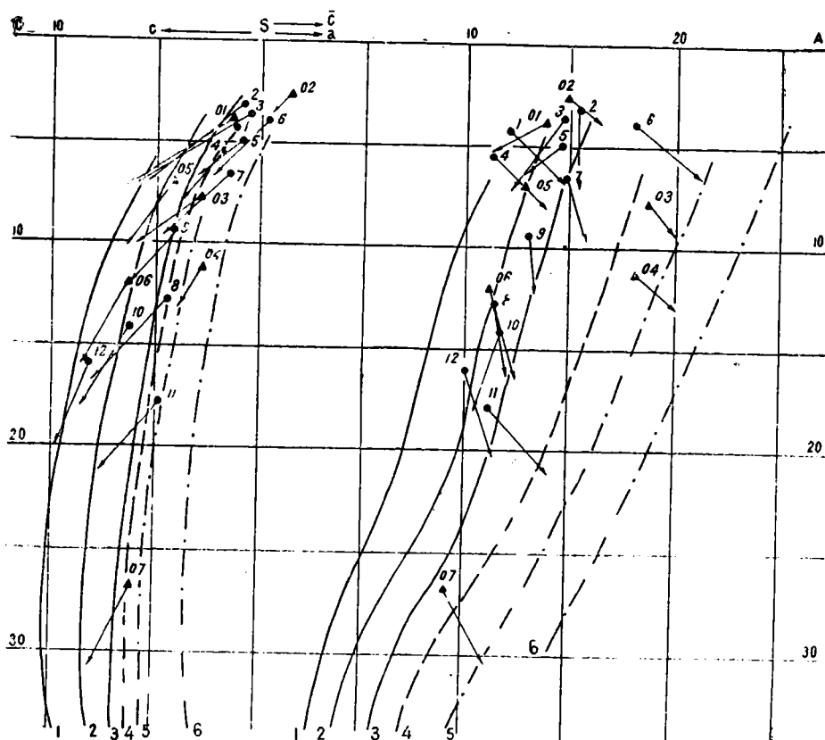
Рис. V—6. Петрохимическая диаграмма постнижнетриасовых экструзивных пород.
