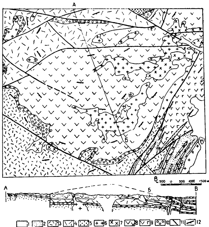
Рис. III—10. Схема геологического строения Ташкумырсайского вулкана. 1 — кайнозойские отложения Илийской депрессии; 2 — вулканогенно-терригенная фация верхней перми; 3 — существенная игнимбритовая фация верхней перми; 4 — то же, нижней перми; 5 — вулканогенно-терригенная фация верхнего карбона; 6—9 — жерловые и околожерловые фации; 6 — neck и экструзии фельзитов, липаритов, микрогранитов; 7 — то же, андезитов и андезито-базальтов; 8 — потоки и покровы андезитов в переслаивании с туфами Ташкумырсайского стратовулкана, 9 — то же, Кызылчекинского стратовулкана; 10 — базальные конгломераты; 11 — разломы; 12 — элементы залегания.
