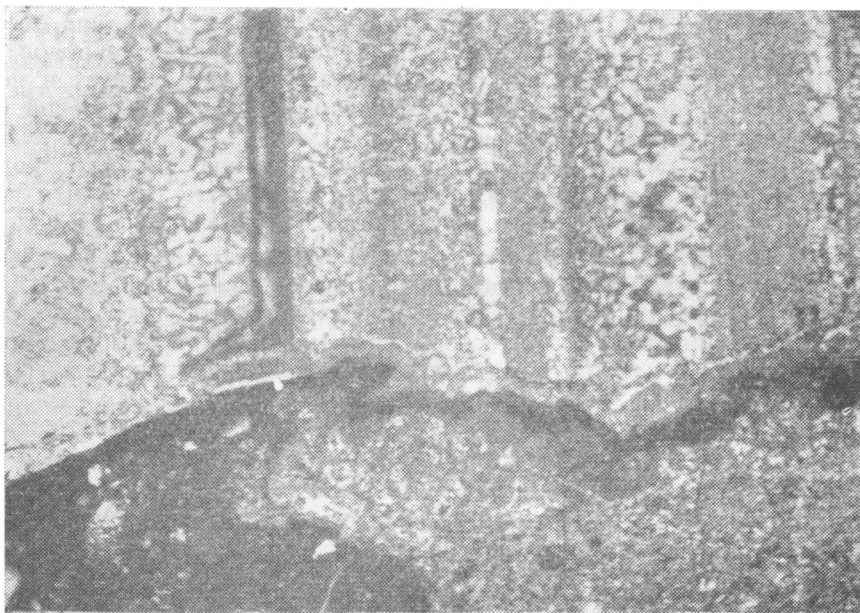
Рис. IV—14. Игнимбрит айнабулакского типа. Ядро шара из полосчатого гидротермального кварца. Ув. 22, при скрещенных николях.
