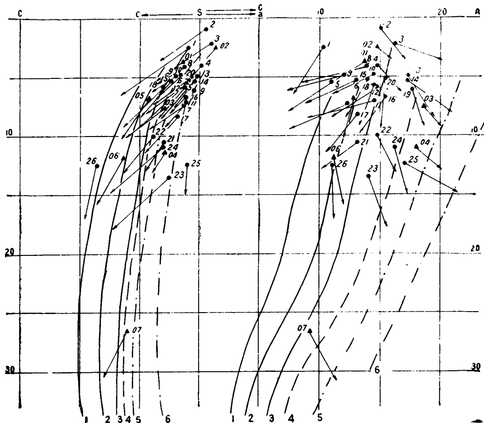
Рис. V—3. Петрохимическая диаграмма верхнепермских эффузивных пород
