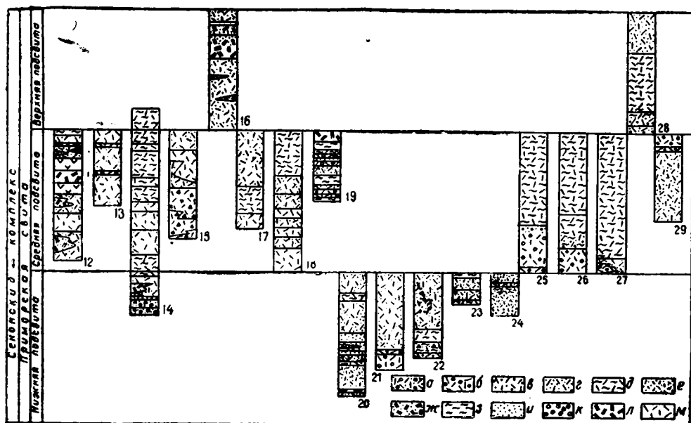
Рис. XI—4. Схема сопоставления разрезов сенонского комплекса. (а—г) — туфы кварцевых порфиров, липаритов, б — агломератовые, в — псефитовые, г — псаммитовые, д — игнимбиты, е — туфопесчаники, ж — туфы дацитов, з — алевриты, и — песчаники, к — конгломераты, л — дациты, м — липариты. Разрезы: 12 — склон Ванчинского вулкана (Чех, 1964), 13 — верховья р. Ванчин (Исполинов, 1963), 14 — склон вулкана Чуматогоу (Дыкин, 1964), 15 — кальдеры вулкана Барачного (Рыбалко, 1964), 16 — правобережье реки Гуэвой (Рыбалко, 1969), 17 — сводный разрез Ольгинского вулкана (Рыбалко, 1969), 18 — С — В бухты Тадуши (Быковская, 1956), 19 — падь Корейская (Быковская, 1956, Рыбалко, 1969), 20 — западное ограничение вулкана Бринера (Рыбалко, 1969), 21 — левобережье Малой Синанчи (Ветренников, 1965), 22 — мыс Якубовского (Ветренников, 1965), 23 — водораздел рек Иодзыхе и Ветроудуй (Ветренников, 1965), 24 — водораздел рек Ветроудуй и Широкий Луг (Ветренников, 1965), 25 — юго-восточное крыло Пластунской впадины (Ветренников, 1965), 26 — северо-западное крыло Пластунской впадины (Ветренников, 1965), 27 — р. Ветроудуй (Ветренников, 1965), 28 — правобережье Малой Синанчи (Ветренников, 1965), 29 — левобережье Малой Синанчи (Ветренников, 1965).
