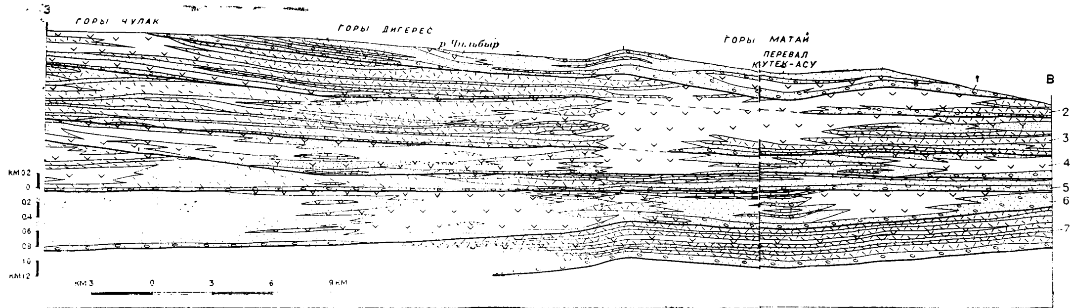
Рис. II—8. Схема фациальной изменчивости средне-верхнепалеозойских вулканогенных свит Южной Джунгарии. Западная часть региона: 1 — достарская свита; 2 — кузгунская свита; 3 — катутауская свита; 4 — конуроленская свита; 5 — айшабулакская свита; 6 — долаптауская свита; 7 — куарасанская свита. (Условные обозначения на рис. II—2).
