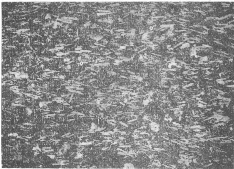
Рис. IV—28. Андезито-базальт с пилотакситовой структурой основной массы. Ув. 22, при скрещенных николях.
