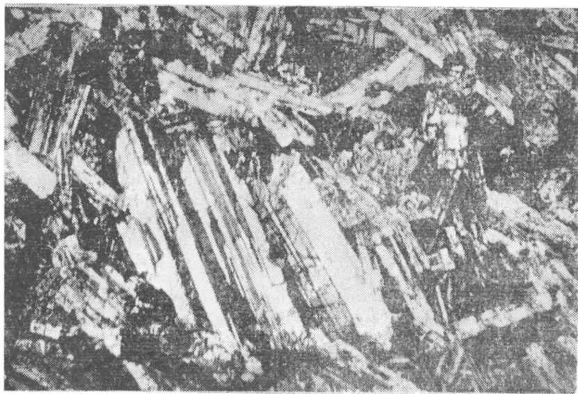
Рис. IV—44. Диорит с субофитовой структурой. Ув. 22, при скрещенных николях.
