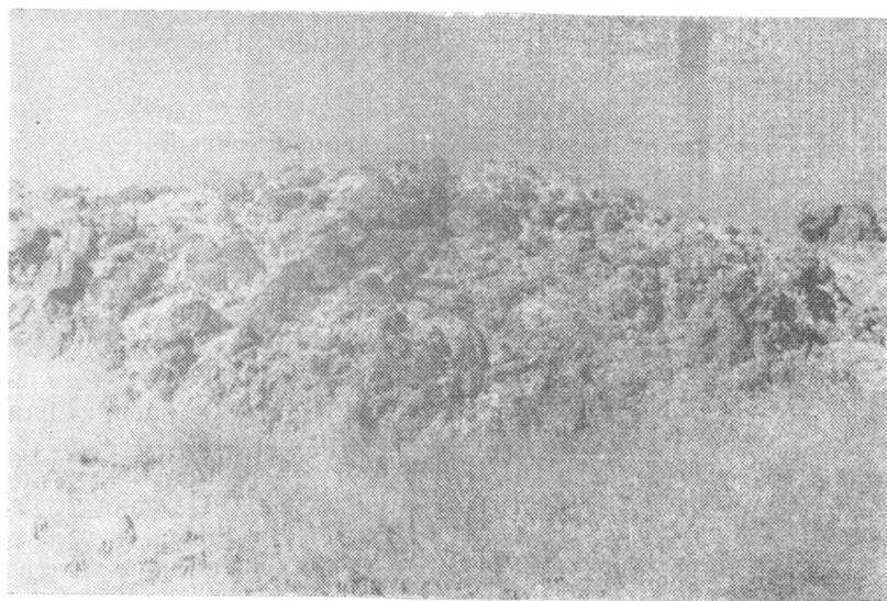
Рис. III—26. Лавобрекчии фельзитов вокруг некка Кызылчеку в горах Архарлы
