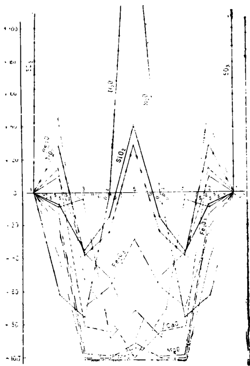
Рис. VI—10. Вариационная диаграмма «привнос — вынос» при метасоматической зональности кызылчекинского типа (к таблице VI—3).
