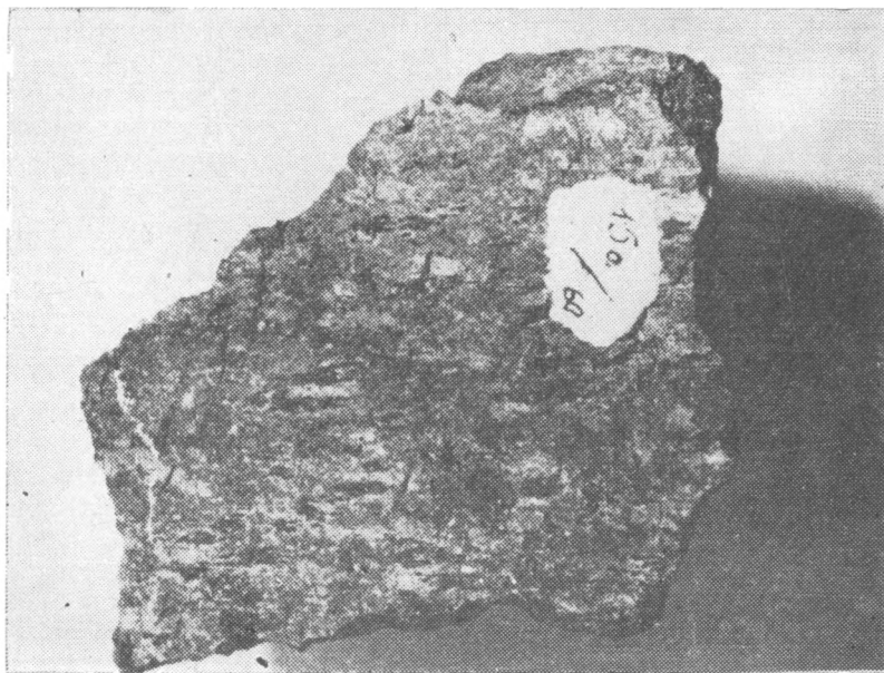
Рис. IV—4. Стекловатый игнимбрид архарлинского типа. Фьямме из черного стекла. 3/4 натур. величины.
