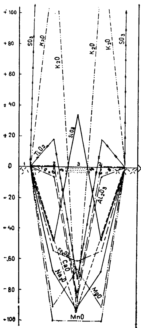
Рис. VI—9. Вариационная диаграмма «привнос — вынос» при метасоматической зональности типа «Скорпион» (к таблице VI—2).
