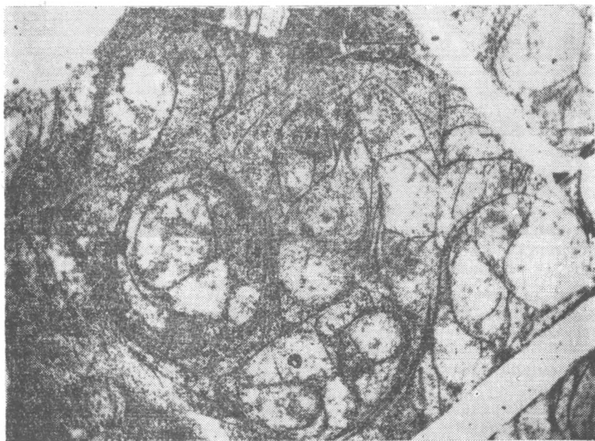
Рис. IV—33. Перлит с перлитовой микроотдельностью. Ув. 22, при одном николе.
