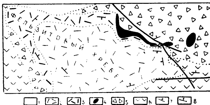
Рис. III—27. Схема геологического строения северной части Северовосто-чного некка в горах Архалы.
