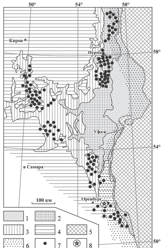
Рис. 1. Положение района работ на схеме распространения рудопоявлений в пермских медистых песчаниках Приуралья по [Харитонов, 2011], с изменениями.
