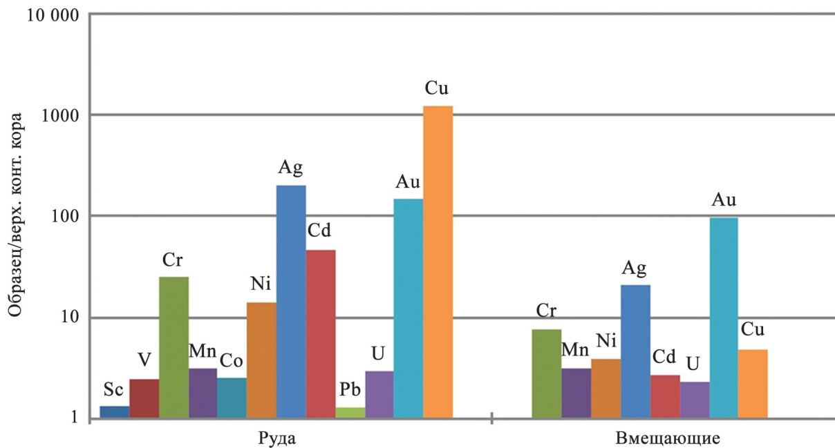
Рис. 4. Распределение микроэлементов (средние значения), нормированных по верхней коре [Тейлор, Мак-Леннан, 1988], в пробах медистых песчаников и вмещающих пород Оренбургского Предураля.
