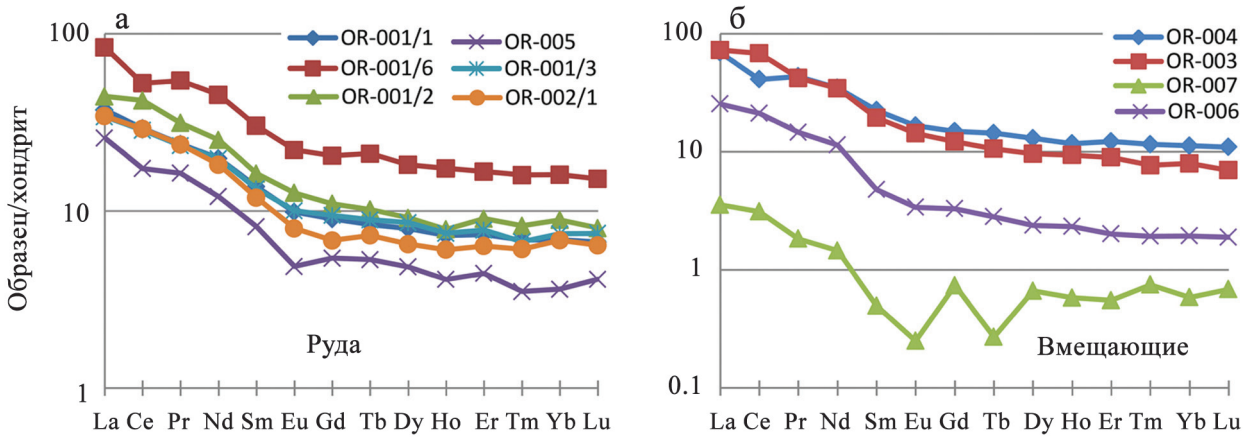
Рис. 5. Распределение РЗЭ, нормированных по хондриту [McDonough, Sun, 1995], в пробах медистых песчаников и вмещающих пород Оренбургского Предуралья.
